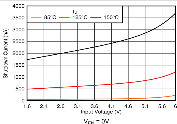
图 5-7. 关断电流与 V_{IN} 间的关系
