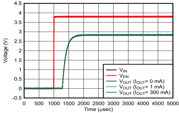
图 5-37. 启动
