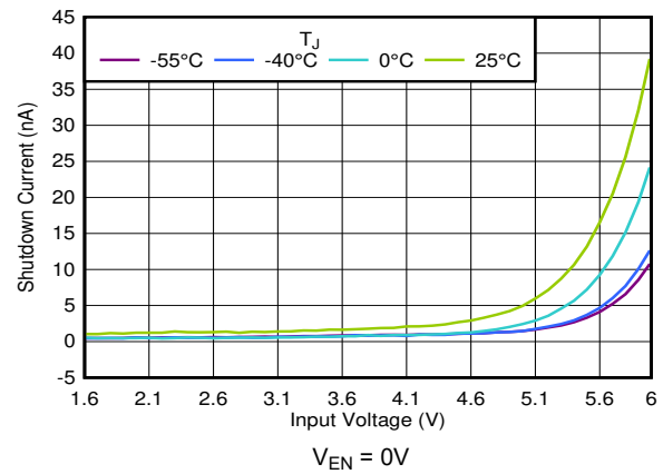
图 5-6. 关断电流与 V_{IN} 间的关系
