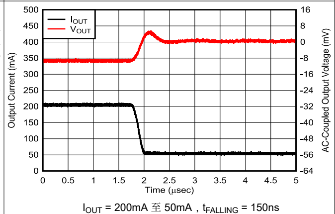
图 5-18. 负载瞬态
