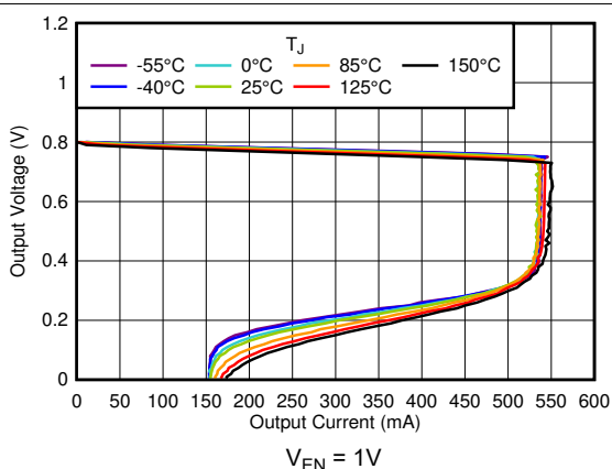
图 5-9. 电流限制
