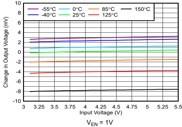
图 5-1. 线路调整率
