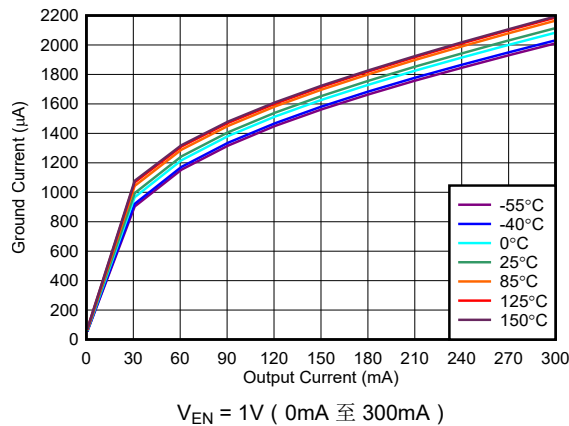
图 5-5. I_{GND} 与 I_{OUT} 间的关系
