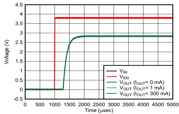
图 7-5. 启动
