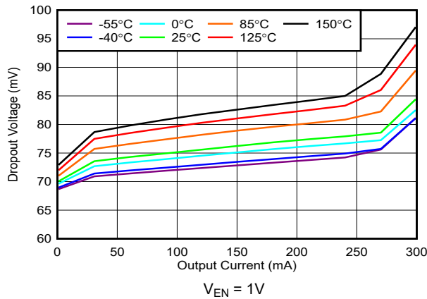
图 5-3. 压降与 I_{OUT} 间的关系
