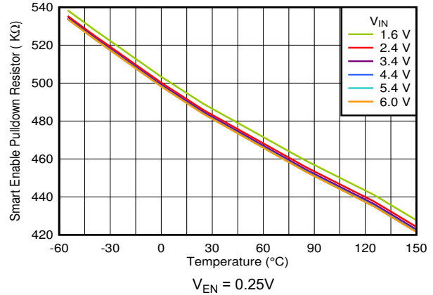
图 5-14. 智能使能下拉电阻与温度和 V_{IN} 间的关系
