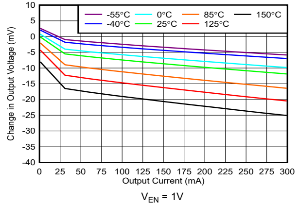
图 5-2. 负载调整率
