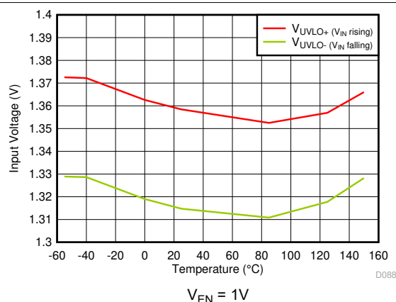
图 5-10. UVLO 阈值与温度间的关系
