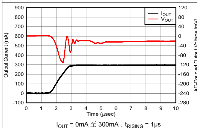
图 5-23. 负载瞬态
