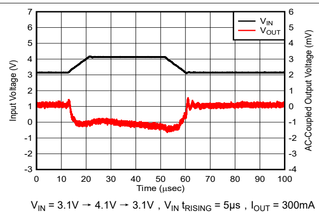
图 5-28. 线路瞬态
