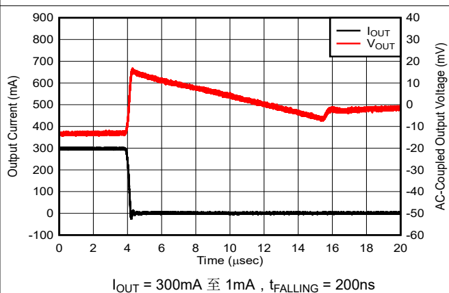
图 5-22. 负载瞬态
