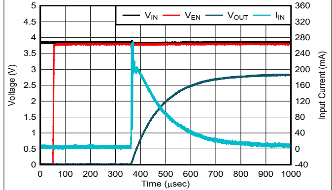
图 5-38. 启动
