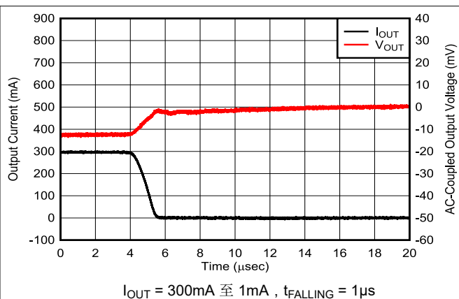
图 5-20. 负载瞬态
