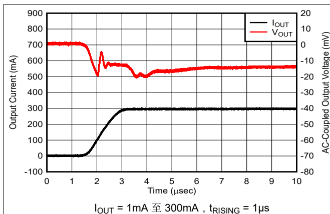
图 5-19. 负载瞬态
