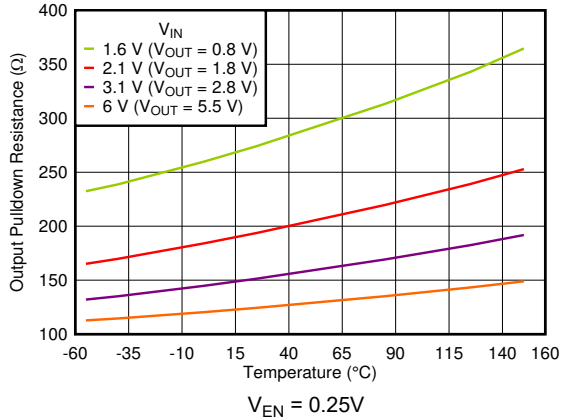
图 5-13. 输出下拉电阻与温度间的关系
