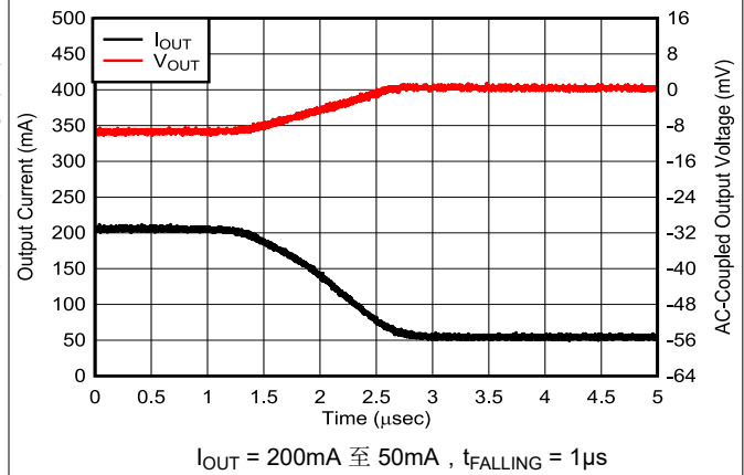
图 5-16. 负载瞬态
