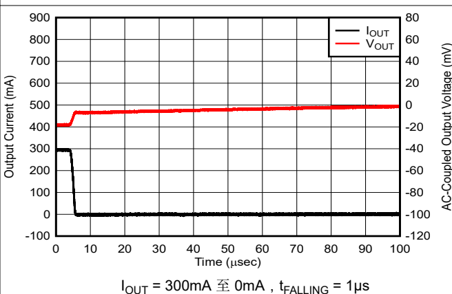
图 5-24. 负载瞬态
