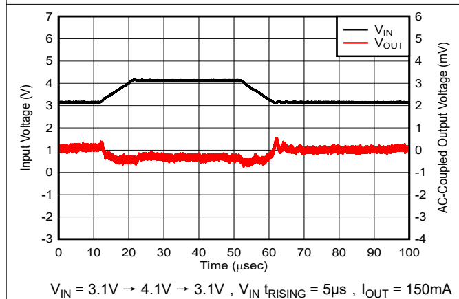
图 5-27. 线路瞬态
