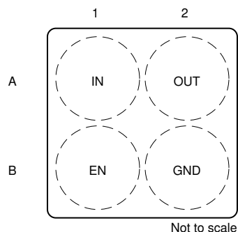
图 4-1. YCK 封装， 4 引脚 DSBGA（顶视图）
