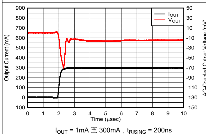
图 5-21. 负载瞬态
