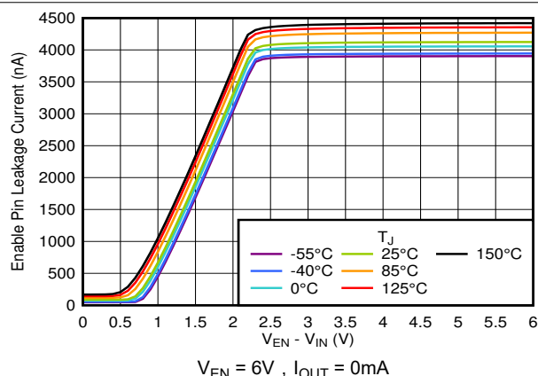
图 5-8. 使能引脚漏电流与 V_{EN} - V_{IN} 间的关系
