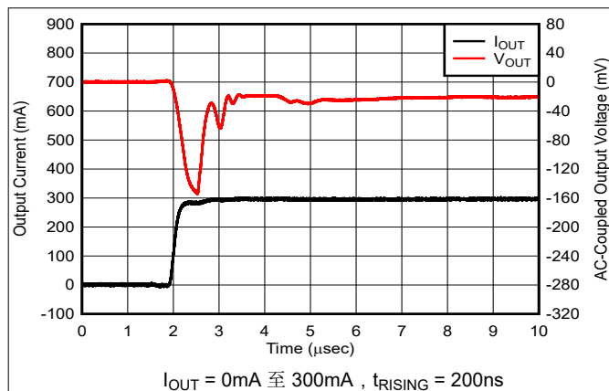
图 5-25. 负载瞬态
