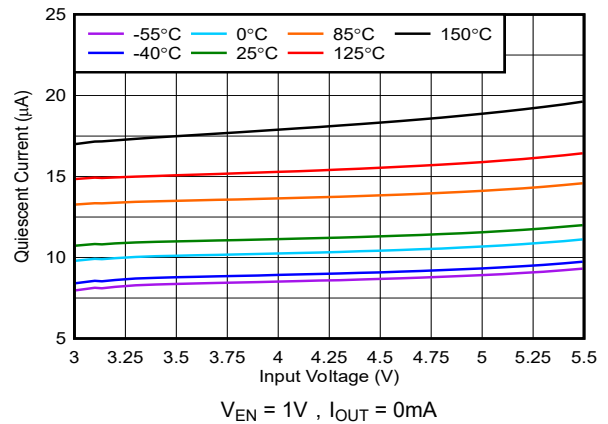
图 5-4. I_{GND} 与 V_{IN} 间的关系
