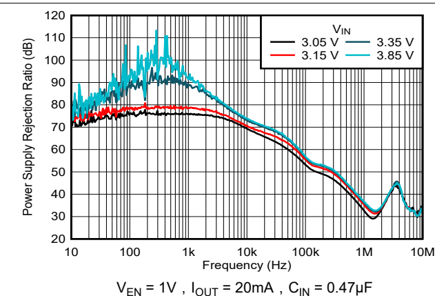
图 5-30. PSRR 与频率和 V_{IN} 间的关系
