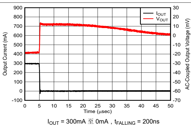
图 5-26. 负载瞬态
