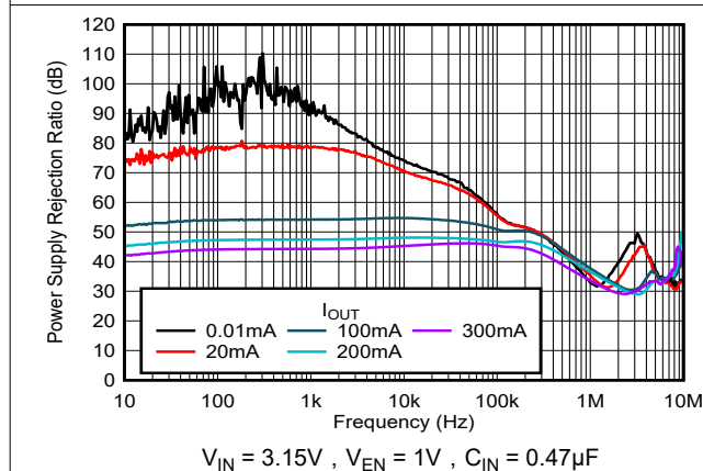
图 5-29. PSRR 与频率和 I_{OUT} 间的关系
