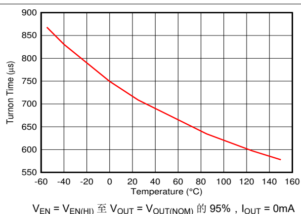
图 5-36. 启动开通时间
