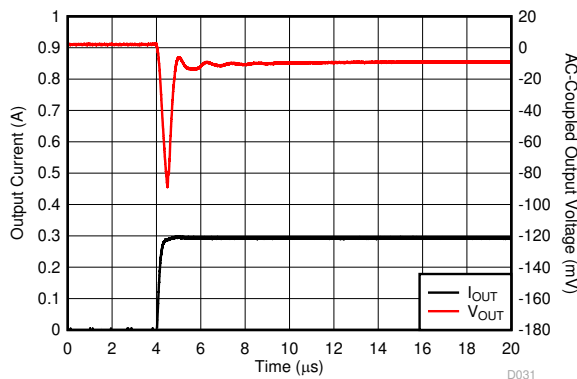
图 5-51. Load Transient
