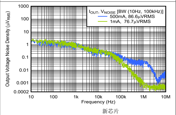
图 5-8. TPS795 输出频谱噪声密度与频率间的关系
