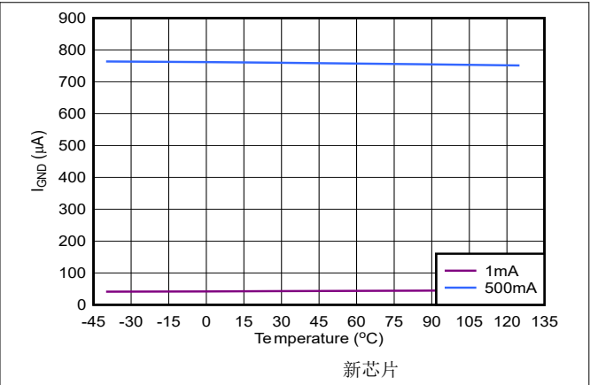
图 5-6. TPS795 接地电流与结温间的关系
