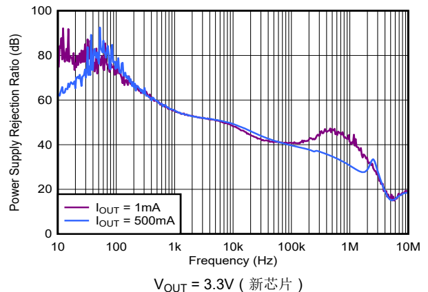
图 5-16. TPS795 波纹抑制与频率
