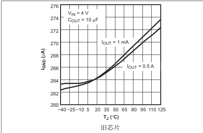
图 5-5. TPS795 接地电流与结温间的关系
