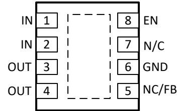
图 4-2. DRB 封装，8 引脚 VSON (顶视图，新芯片)
