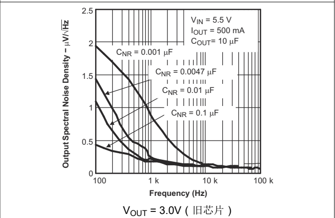
图 5-10. TPS795 输出频谱噪声密度与频率间的关系
