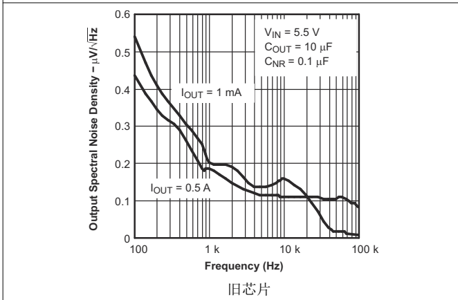
图 5-9. TPS79530 输出频谱噪声密度与频率间的关系
