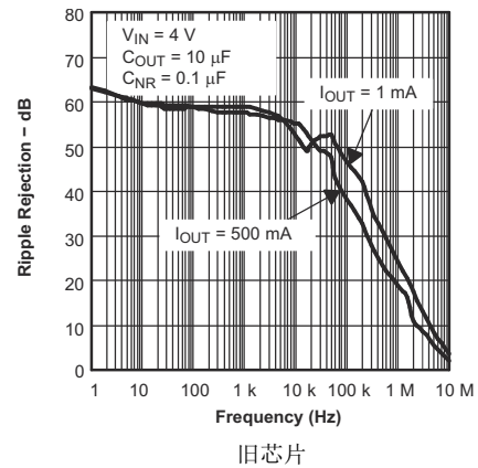
图 5-14. TPS795 波纹抑制与频率
