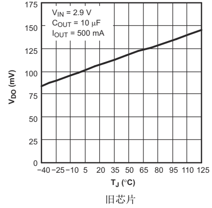
图 5-12. TPS795 压降电压与结温间的关系
