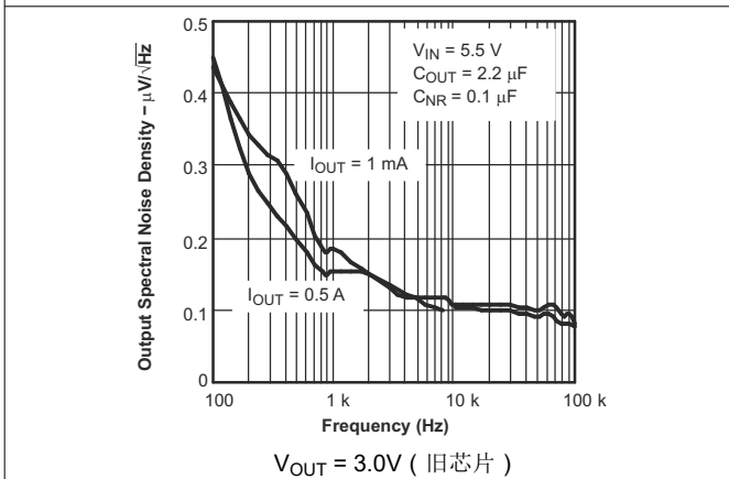
图 5-7. TPS795 输出频谱噪声密度与频率间的关系
