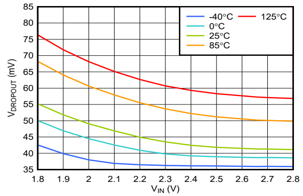
新芯片, I_{OUT} = 200\text{mA}
