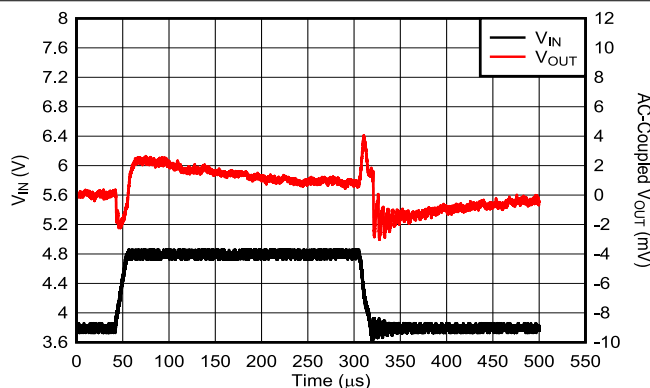
图 5-24. TPS793 线路瞬态响应
