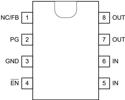
图 4-1. D Package, 8-Pin SOIC (Top View)
