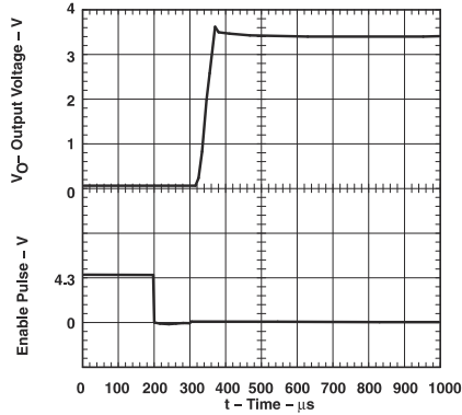
图 7-10. TPS76633 Output Voltage vs Time (Legacy Chip)
