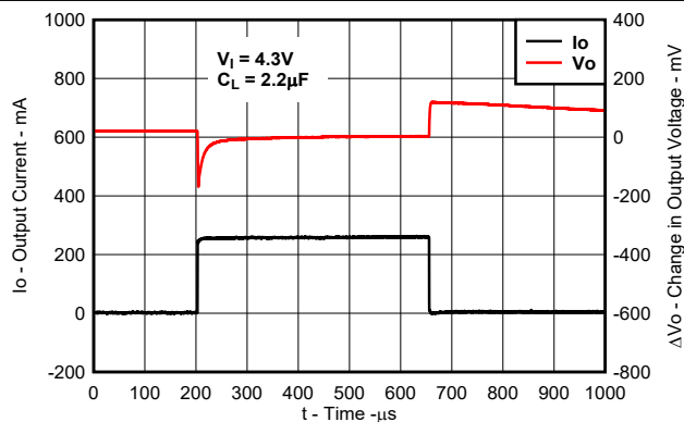
图 7-7. TPS76633 Load Transient Response (Legacy Chip)
