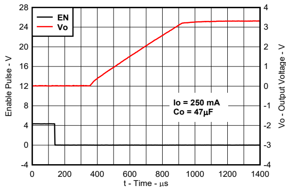
图 7-10. TPS76633 Output Voltage vs Time (Legacy Chip)
