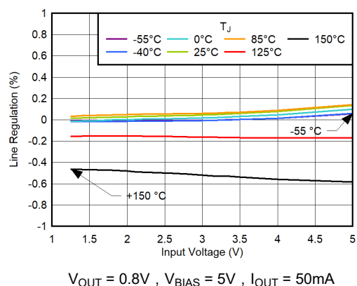
图 5-15. 线性调整率与输入电压间的关系
