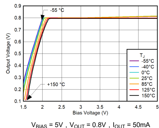
图 5-16. 输出电压与偏置电压间的关系
