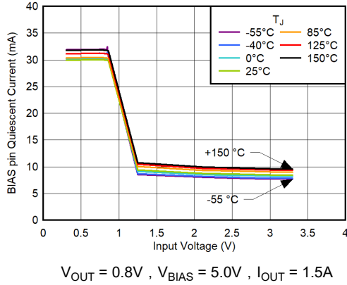
图 5-19. BIAS 引脚静态电流与输入电压之间的关系
