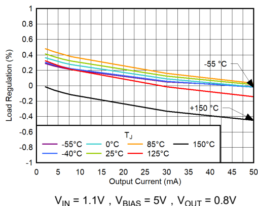
图 5-13. 负载调节与 0mA 至 50mA 输出电流间的关系
