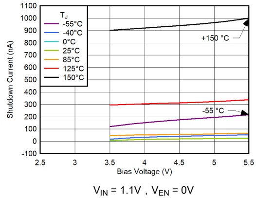
图 5-22. 关断电流（GND 引脚）与偏置电压间的关系
