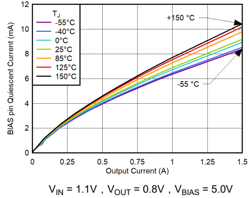
图 5-20. BIAS 引脚静态电流与输出电流间的关系
