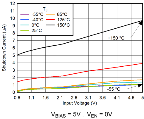
图 5-21. 关断电流（GND 引脚）与输入电压间的关系
