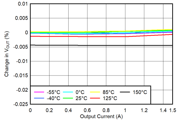
图 5-4. 负载调节 (新芯片)
