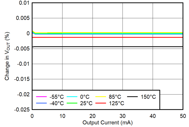
图 5-2. 负载调节 (新芯片)
