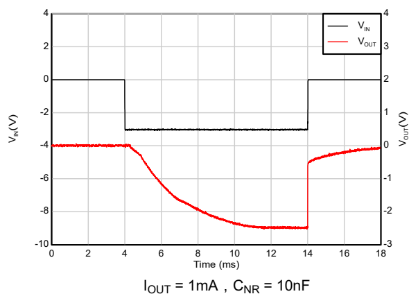
图 5-55. TPS72325 启动响应 ( V_{IN} 和 EN 连接在一起) (新芯片)
