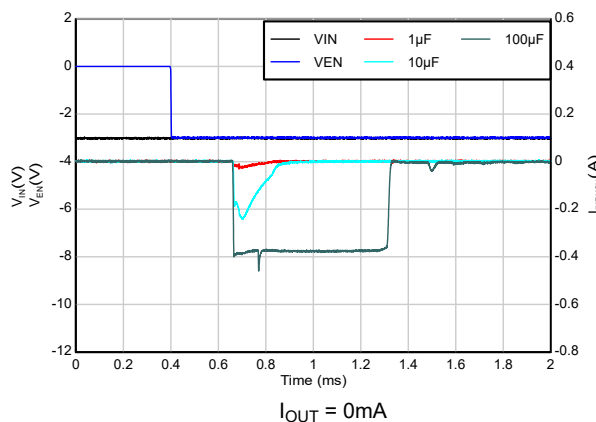
图 5-57. 启动浪涌电流与 C_{OUT} 间的关系 (新芯片)
