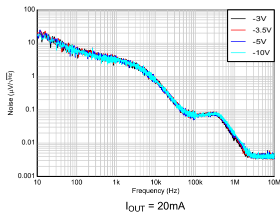
图 5-63. TPS72325 总噪声与 V_{IN} 间的关系 (10Hz 至 10MHz) (新芯片)
