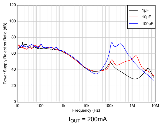
图 5-77. PSRR 与 C_{OUT} 间的关系 (新芯片)
