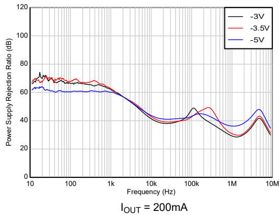
图 5-75. PSRR 与 V_{IN} 间的关系 (新芯片)
