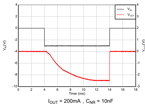
图 5-56. TPS72325 启动响应 ( V_{IN} 和 EN 连接在一起) (新芯片)
