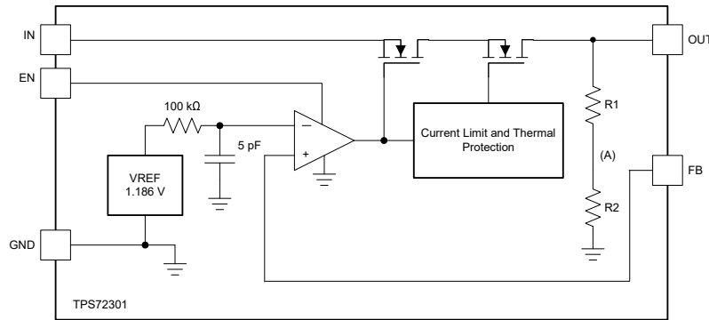
图 6-1. 功能方框图（可调，旧芯片）
