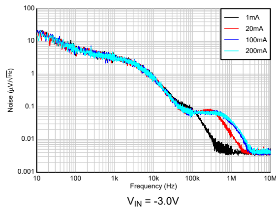
图 5-61. TPS72325 总噪声与 I_{OUT} 间的关系 (10Hz 至 10MHz) (新芯片)
