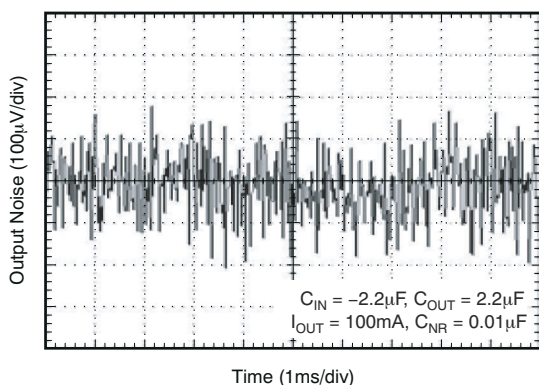
图 5-67. TPS72325 输出噪声与时间间的关系 (旧芯片)
