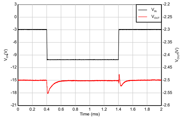
图 5-37. TPS72325 线路瞬态响应 (新芯片)
