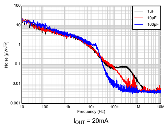
图 5-65. TPS72325 总噪声与 C_{OUT} 间的关系 (10Hz 至 10MHz) (新芯片)
