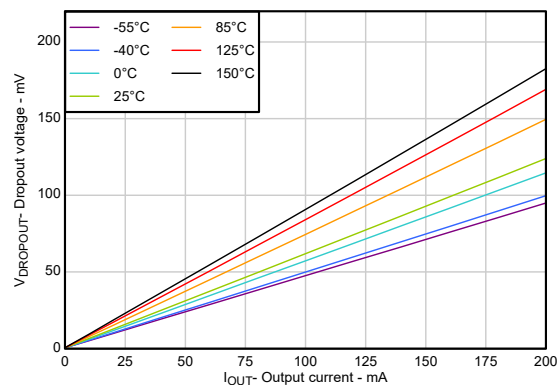
图 5-8. 压降电压与输出电流间的关系 (新芯片)
