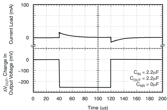
图 5-43. TPS72325 负载瞬态响应 (旧芯片)
