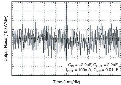
图 7-4. TPS72325 输出噪声与时间的关系 (旧芯片)
