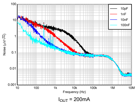
图 5-59. TPS72325 总噪声与 C_{NR} 间的关系 (10Hz 至 10MHz) (新芯片)
