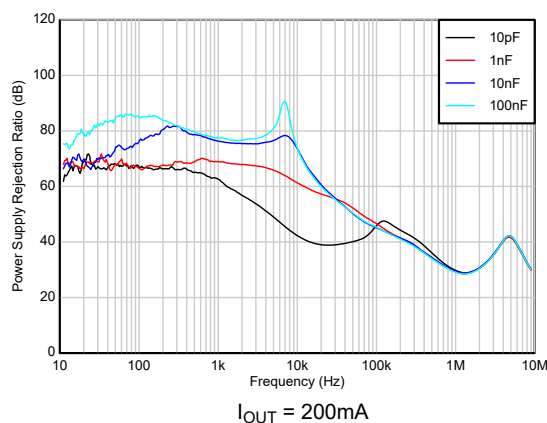
图 5-72. PSRR 与 C_{NR} 间的关系 (新芯片)
