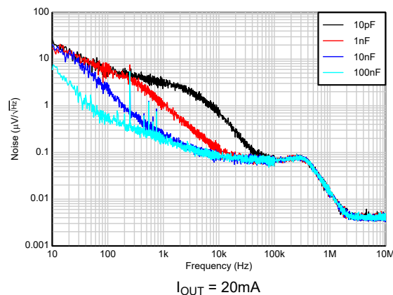
图 5-60. TPS72325 总噪声与 C_{NR} 间的关系 (10Hz 至 10MHz) (新芯片)
