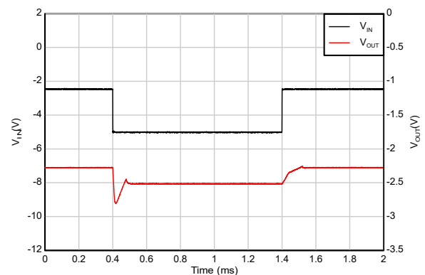
图 5-39. TPS72325 线路瞬态响应 (新芯片)
