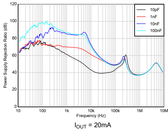
图 5-73. PSRR 与 C_{NR} 间的关系 (新芯片)
