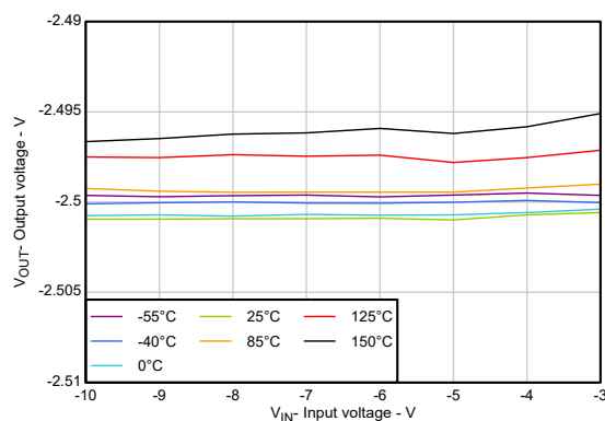
图 5-2. 输出电压与输入电压间的关系 (新芯片)
