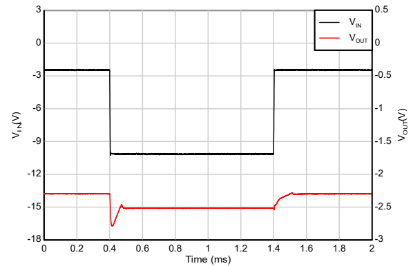
图 5-38. TPS72325 线路瞬态响应 (新芯片)
