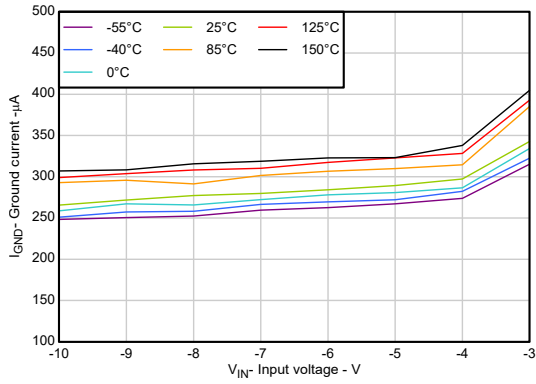
图 5-13. 接地电流与输入电压间的关系 (新芯片)
