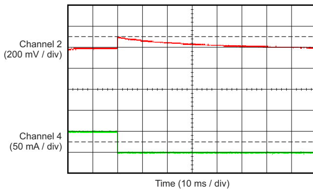
图 5-27. TPS70912-Q1 负载瞬态 (0mA 至 50mA)
