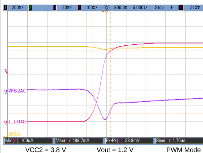
图 7-5. VDD2 Rising Load Transient Response
