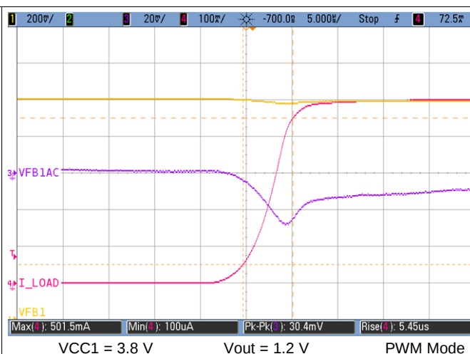
图 7-3. VDD1 Rising Load Transient Response
