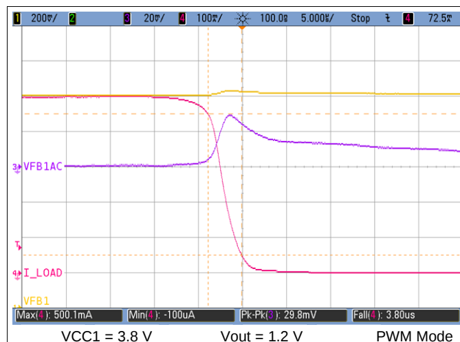
图 7-2. VDD1 Falling Load Transient Response
