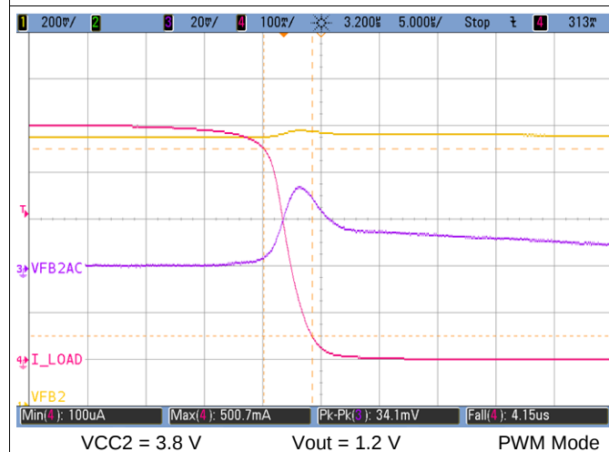
图 7-4. VDD2 Falling Load Transient Response
