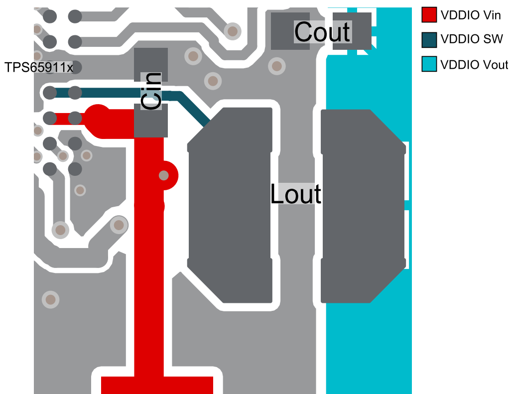
图 7-10. VDDIO Layout
