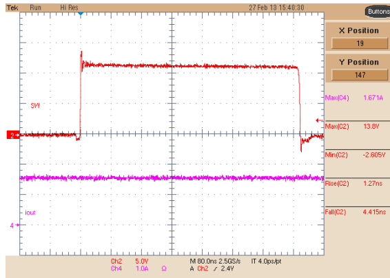
图 8-41. Buck 3 Switching Node, 1.5-A Load
