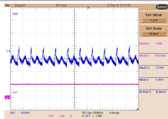
图 8-14. Buck 1 Ripple, 1-A Load
