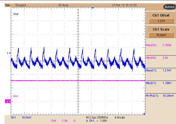
图 8-16. Buck 1 Ripple, 3-A Load
