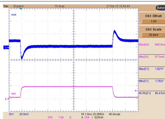
图 8-28. Buck 2 Dynamic Response, 0-A to 1-A Step
