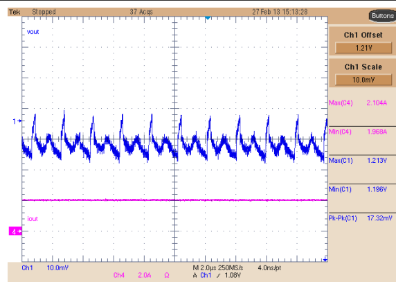
图 8-15. Buck 1 Ripple, 2-A Load
