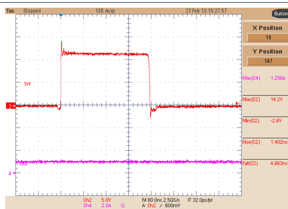
图 8-26. Buck 2 Switching Node, 1-A Load
