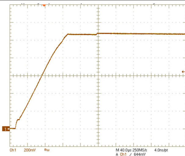
图 8-7. BUCK3 Converter Start-Up
