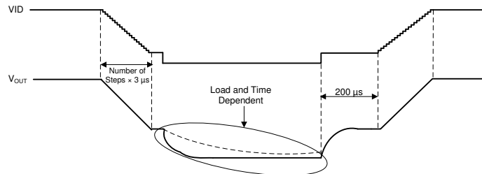
图 7-6. DVS Timing Diagram II
