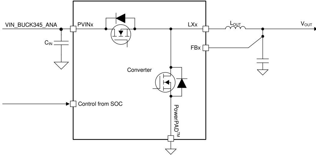
图 8-3. Converter Diagram
