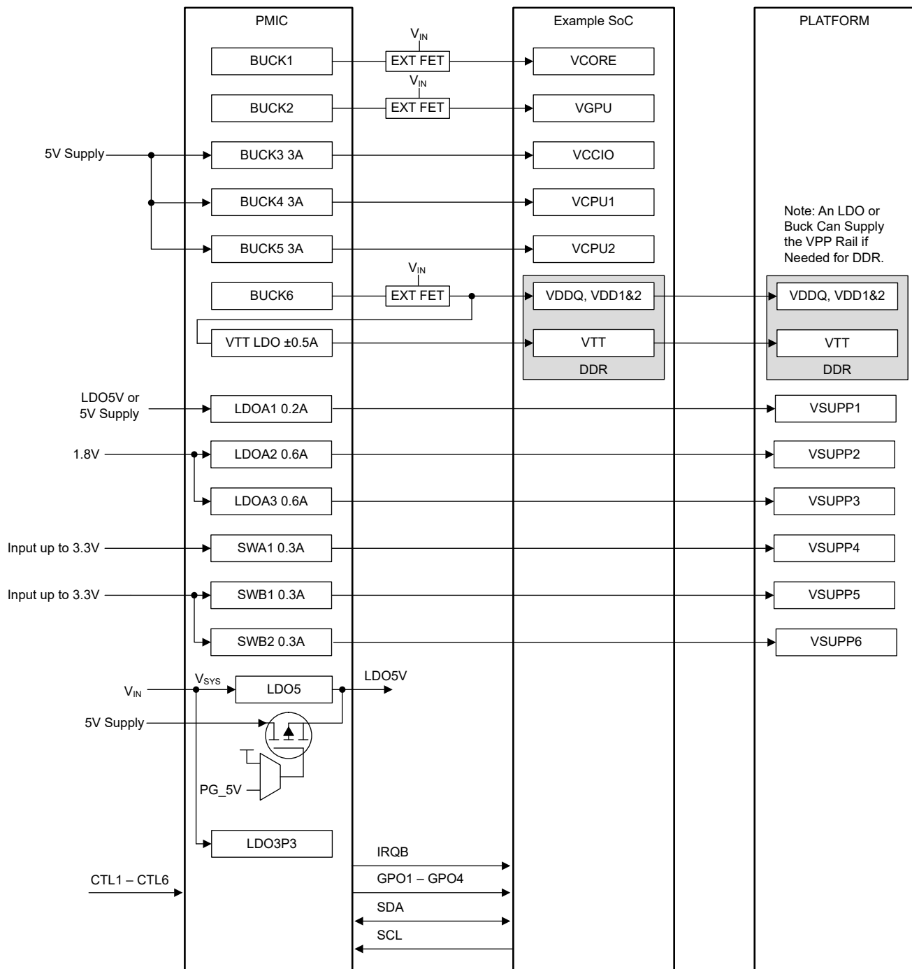
图 6-2. Power Map Example
