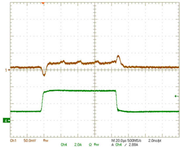
图 7-5. BUCK3 Converter Load Transient
