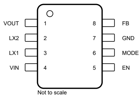
图 4-1. 8 引脚 DRL SOT-5X3 封装 (俯视图)
