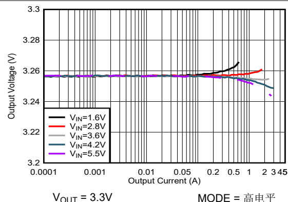
图 7-4. 负载调节 (FPWM)
