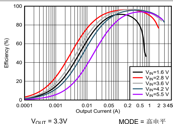
图 7-3. 效率与输出电流间的关系 (FPWM)
