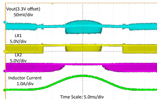
图 7-17. 输入电压为 3.6V 时的负载扫描
