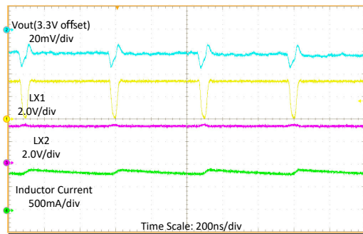
图 7-8. 1A 负载时的开关波形
