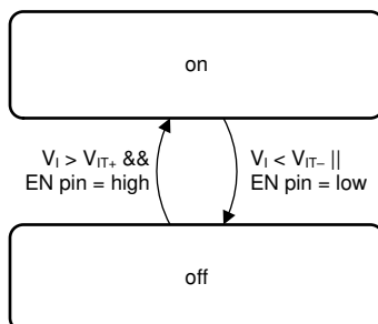
图 6-3. 器件功能模式
