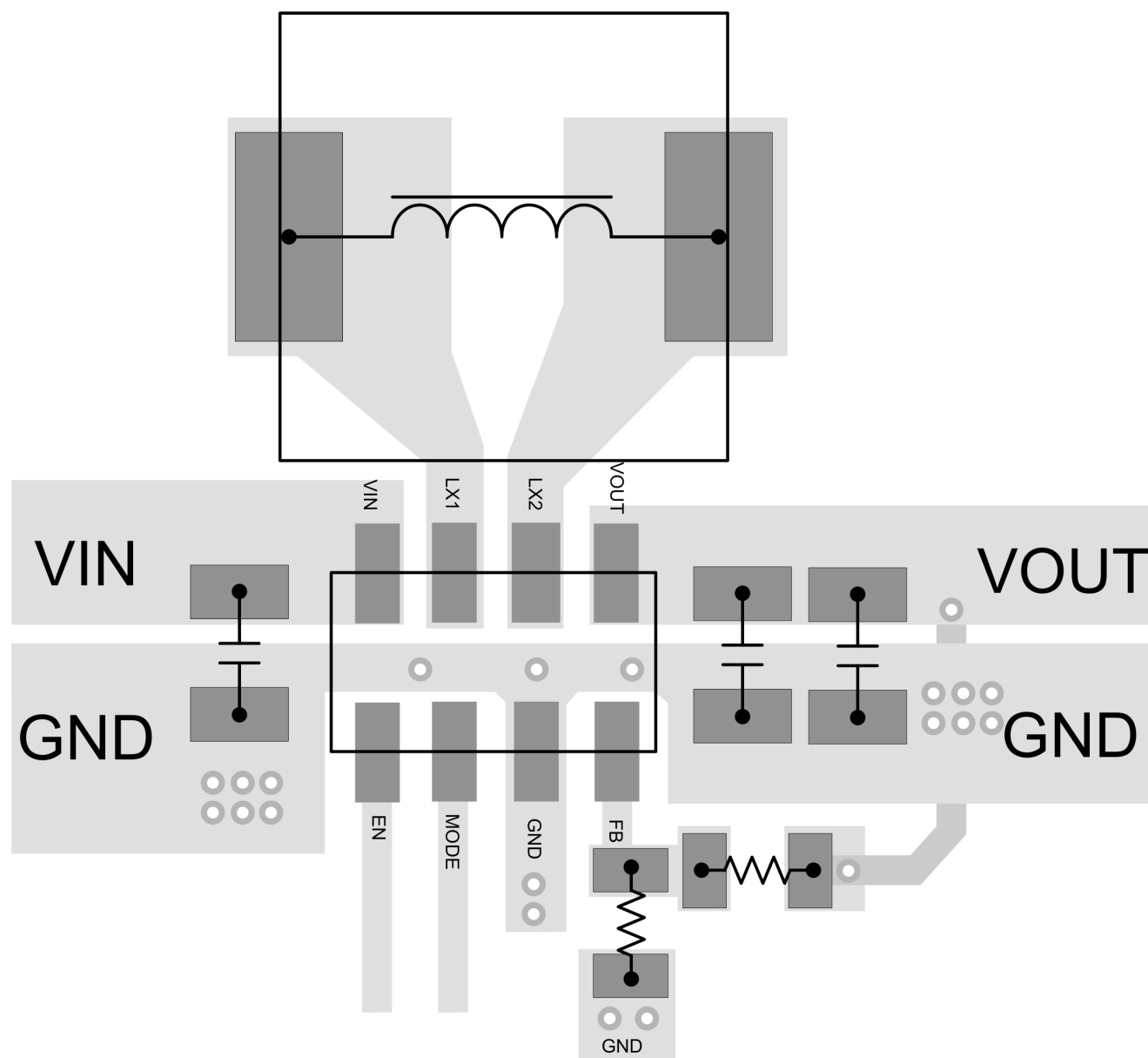
图 7-24. 布局示例
