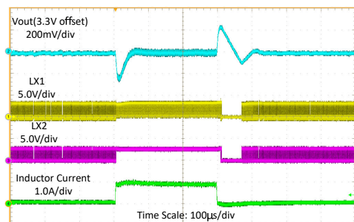
图 7-14. 输入电压为 2.7V 时的负载瞬态
