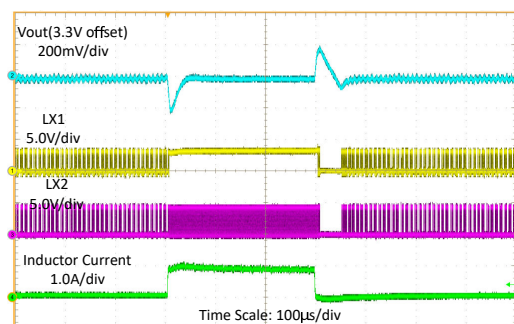
图 7-16. 输入电压为 3.6V 时的负载瞬态
