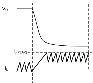
图 6-2. 短路保护期间的典型器件行为
