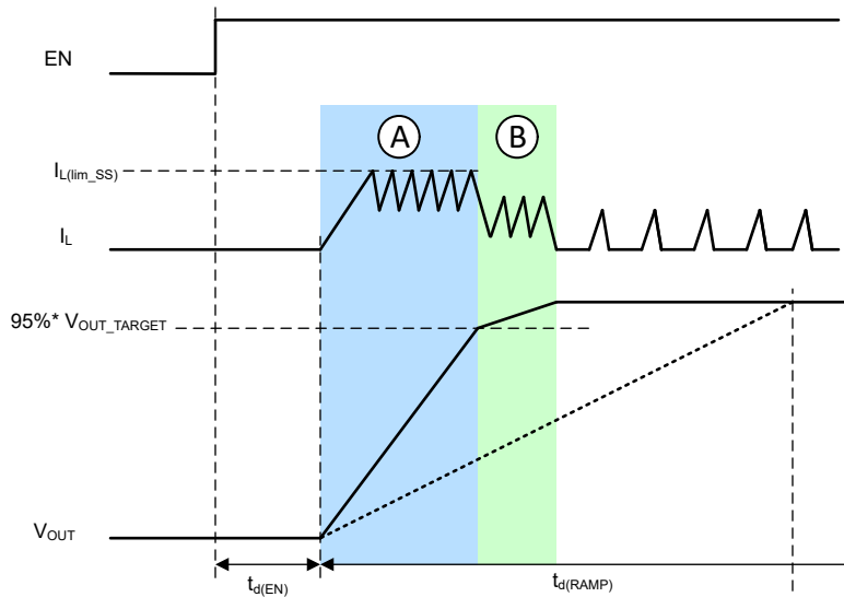
图 6-1. 典型的软启动行为
