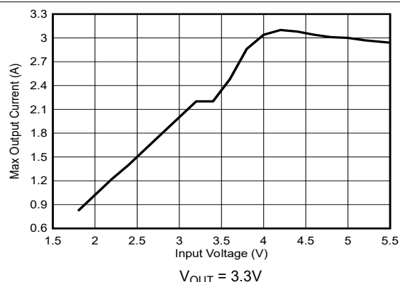
图 7-2. 典型输出电流能力与输入电压间的关系
