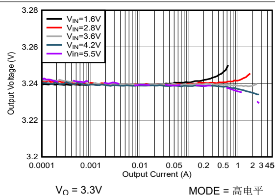
图 7-6. 负载调节 (PFM)
