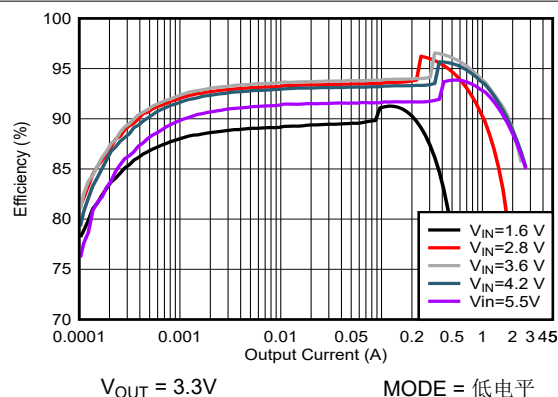
图 7-5. 效率与输入电压间的关系 (PFM)
