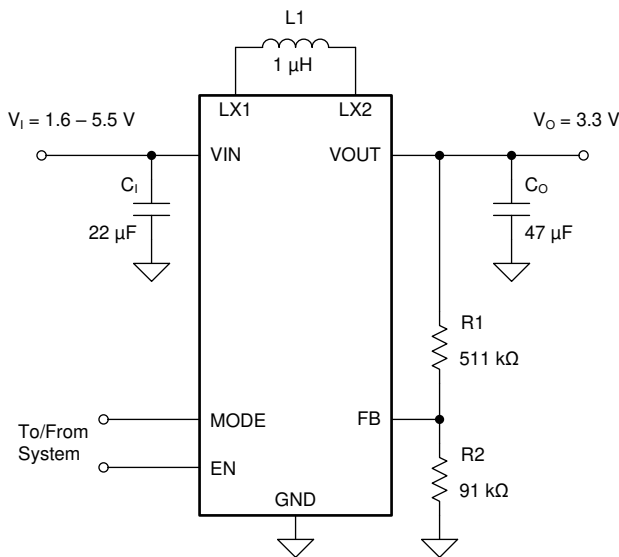
图 7-1. 3.3V OUT 典型应用
