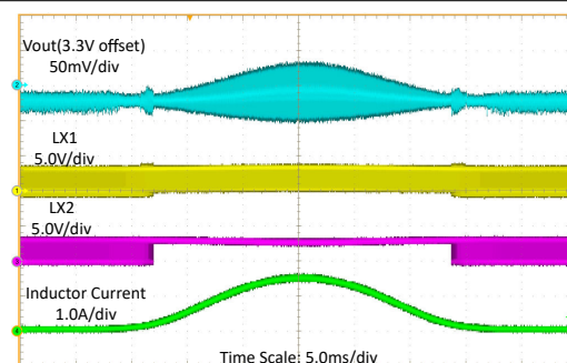
图 7-15. 输入电压为 2.7V 时的负载扫描
