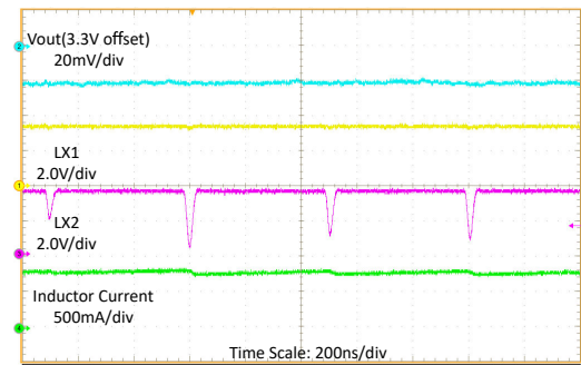
图 7-9. 1A 负载时的开关波形
