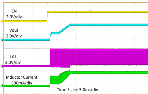
图 7-10. 负载为 1A 并采用降压运行模式时的开关波形
