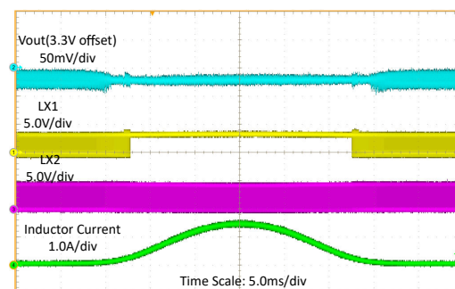
图 7-19. 输入电压为 4.3V 时的负载扫描
