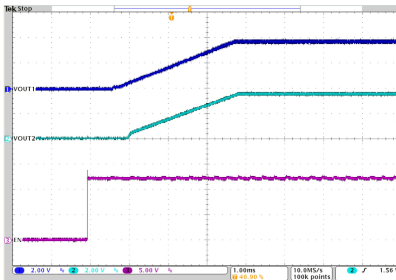
图 9-85. Tracking
