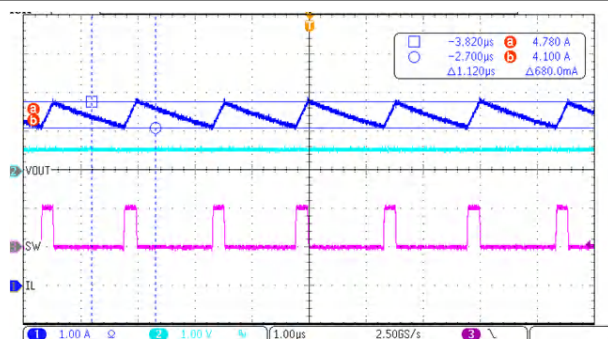
图 9-78. Output Voltage Ripple
