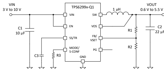
简化原理图
