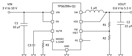
简化原理图
