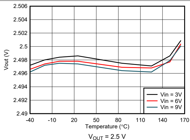
图 7-6. Output Voltage Accuracy - VSET Selected
