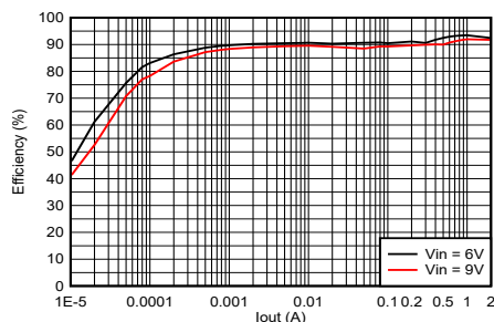
效率与输出电流间的关系 (3.3 V O , 2.5MHz, 1 μH, 自动 PFM 或 PWM)
