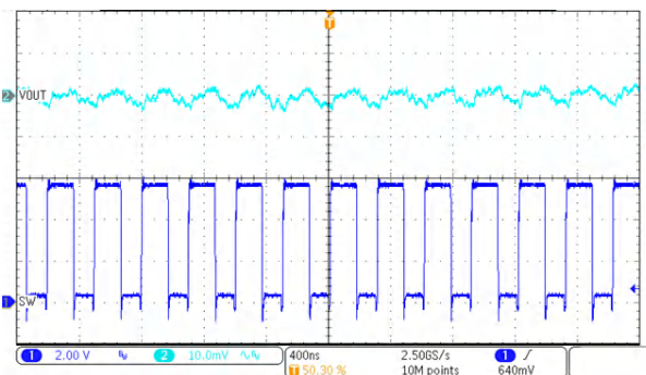
图 9-77. Output Voltage Ripple
