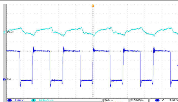
图 9-76. Output Voltage Ripple
