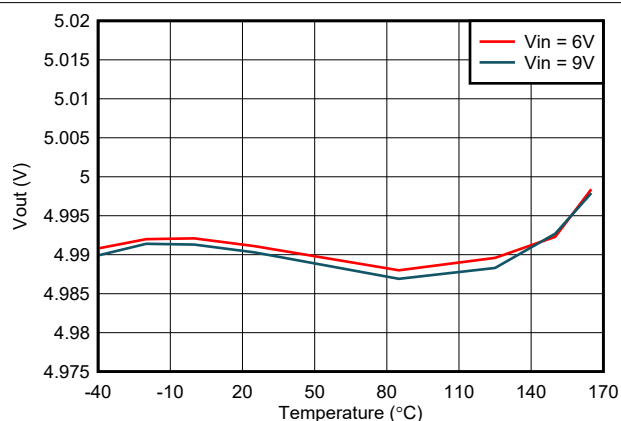
图 7-4. Output Voltage Accuracy - VSET Selected
