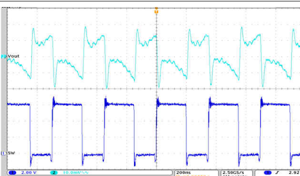
图 9-77. Output Voltage Ripple
