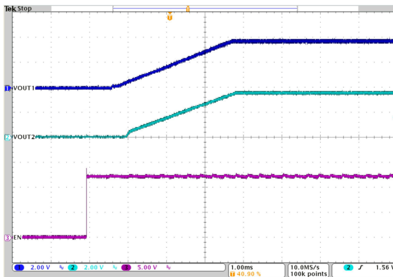
图 9-84. Tracking
