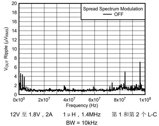
图 5-8. 第 2 个 L-C 滤波器之后的 V_{OUT} 纹波 FFT
