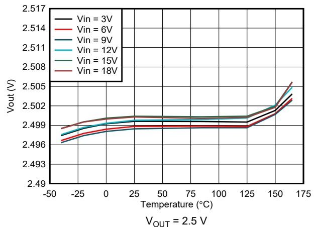
图 7-6. Output Voltage Accuracy - VSET Selected
