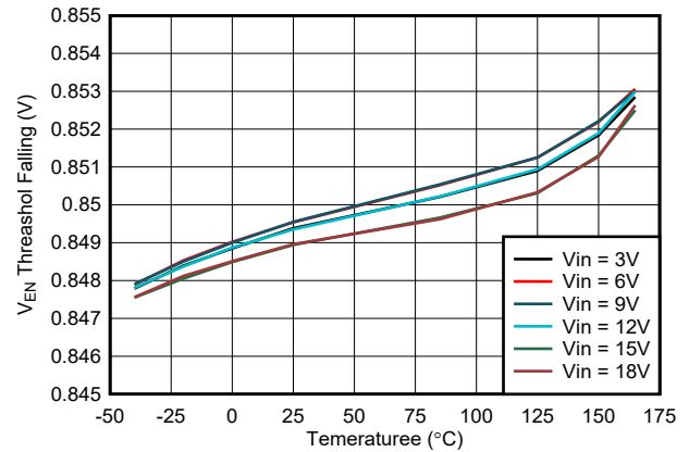
图 7-22. Percise EN Threshold vs Temperature
