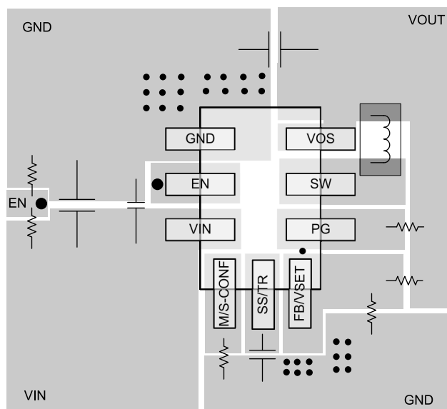
图 9-69. Layout
