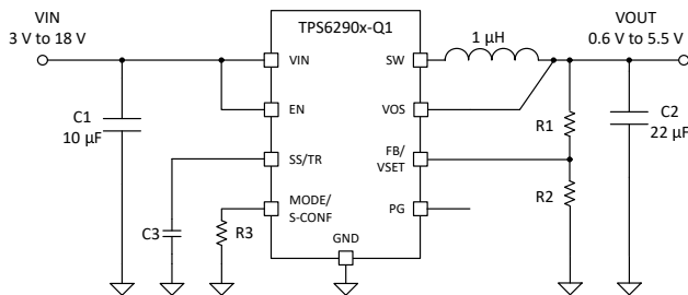
简化原理图
