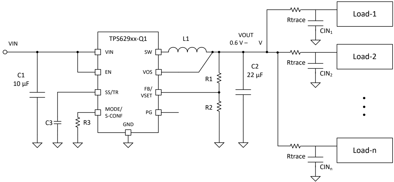
图 9-65. Multiple Loads
