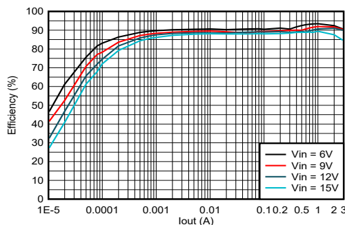
效率与输出电流间的关系 (3.3 V O , 2.5MHz, 1μH, 自动 PFM 或 PWM)
