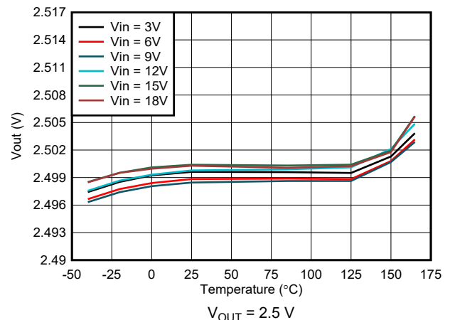
图 7-6. Output Voltage Accuracy - VSET Selected
