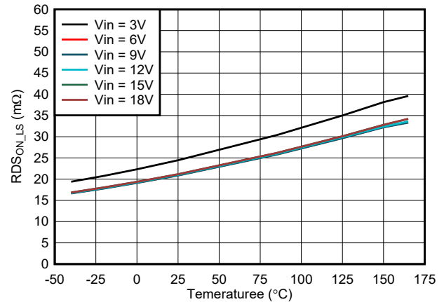
图 7-14. Low Side R_{DS(on)} vs Temperature
