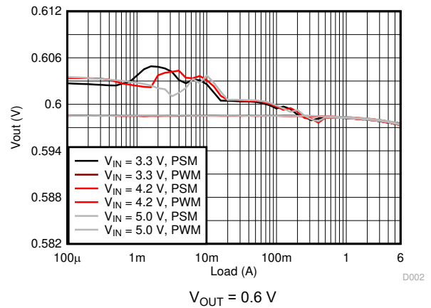
图 9-3. Load Regulation
