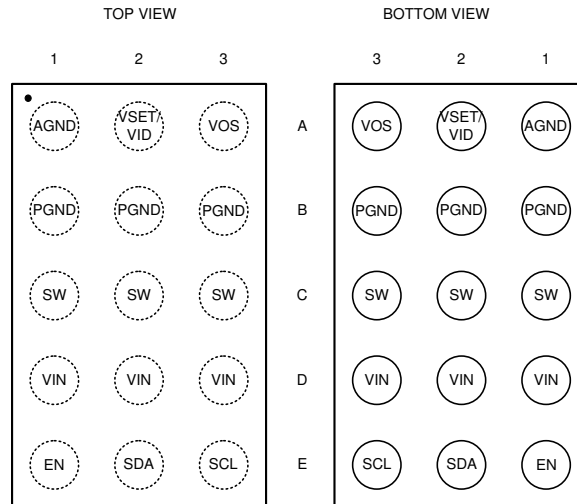
图 6-1. YCG (15 Pin)
