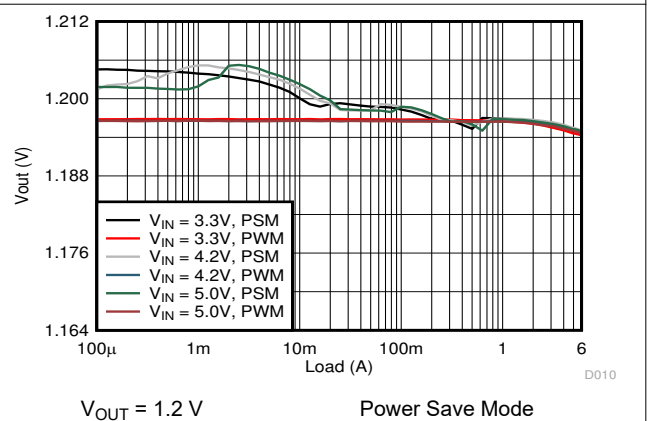
图 9-7. Load Regulation
