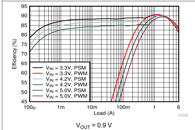
图 9-4. Efficiency
