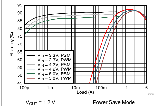
图 9-6. Efficiency
