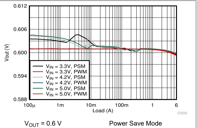
图 9-3. Load Regulation
