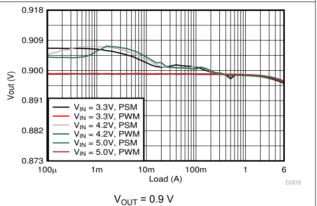
图 9-5. Load Regulation
