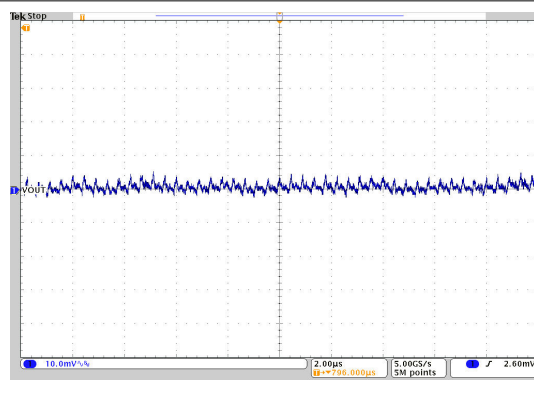
图 10-47. Output Voltage Ripple
