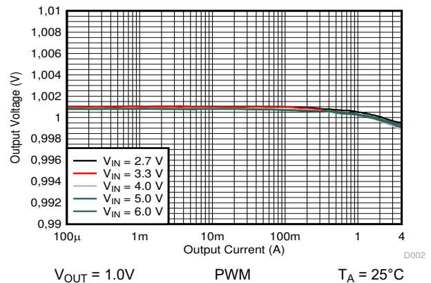
图 9-19. 输出电压与输出电流间的关系
