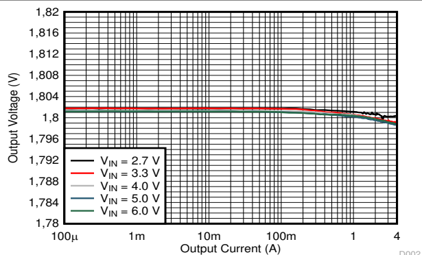
图 9-15. 输出电压与输出电流间的关系
