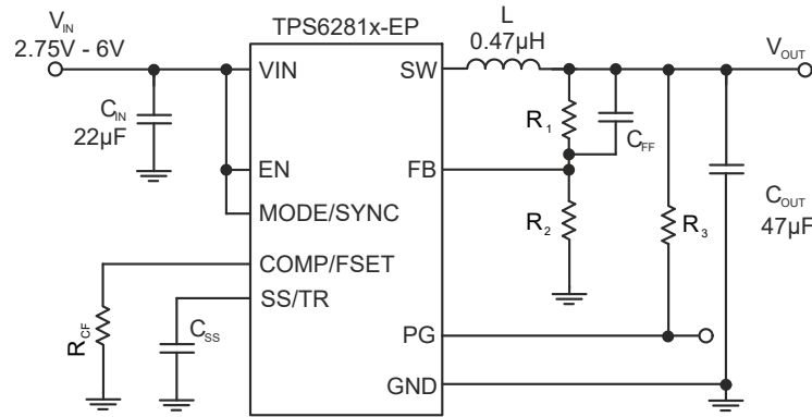
图 9-1. 典型应用
