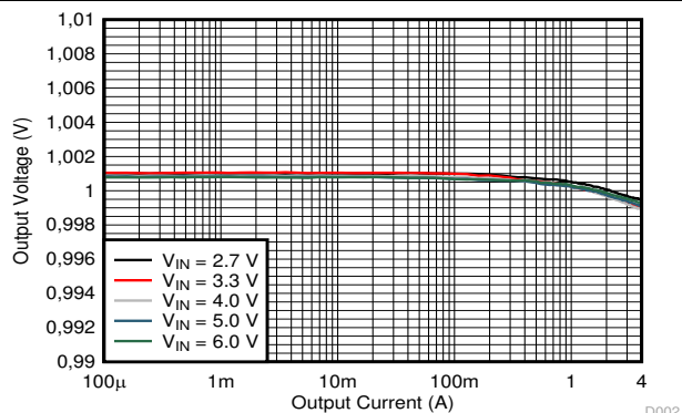
图 9-17. 输出电压与输出电流间的关系
