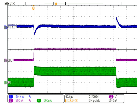
强制 PWM V_{OUT} = 1.2V VSEL/MODE = VIN 模式 (启动后) 上升/下降时间 < 1\mu s I_{OUT} = 5mA 至 500mA
