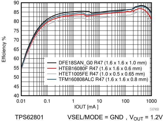
图 8-8. 电感器比较
