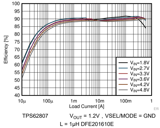
图 8-12. 节能模式效率, V OUT = 1.2V
