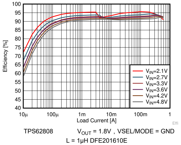
图 8-13. 节能模式效率, V OUT = 1.8V
