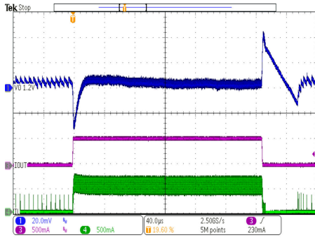
TPS62801 V_{OUT} = 1.2V VSEL/MODE = GND 上升/下降时间 < 1\mu s PFM/PWM 模式 I_{OUT} = 5mA 至 500mA
