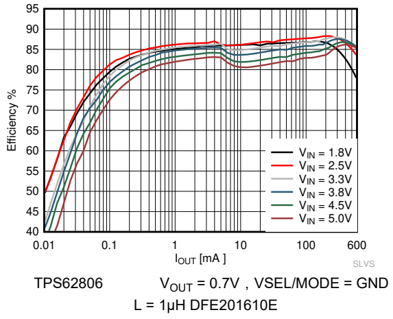
图 8-11. 节能模式效率, V OUT = 0.7V
