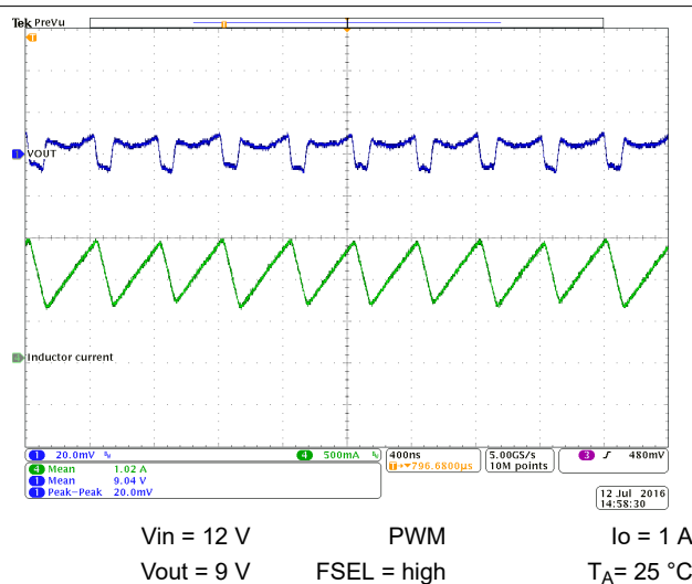
图 10-65. Output Voltage Ripple
