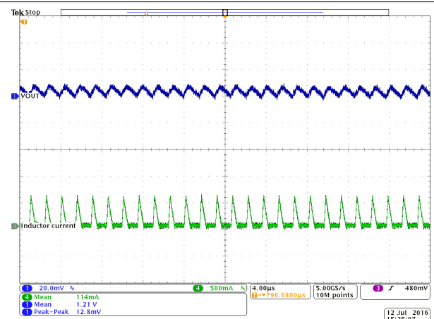
图 10-36. Output Voltage Ripple
