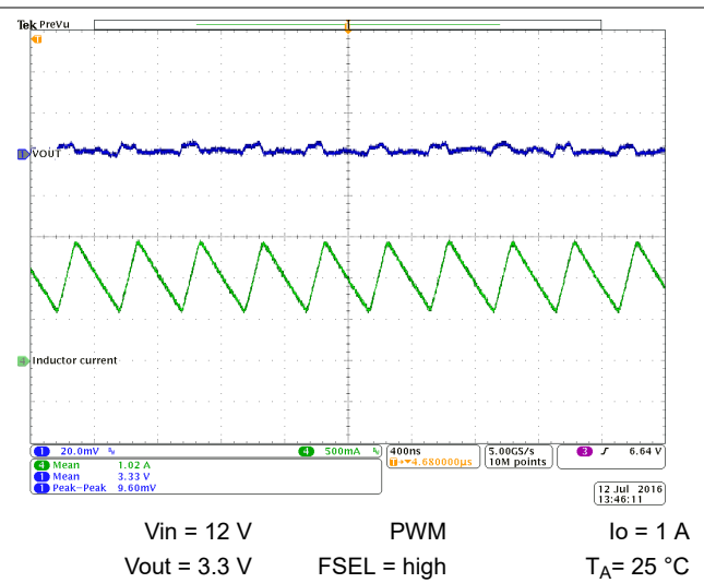
图 10-51. Output Voltage Ripple
