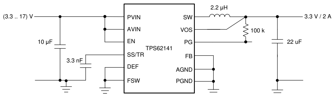
图 9-44. 3.3-V/2-A Power Supply
