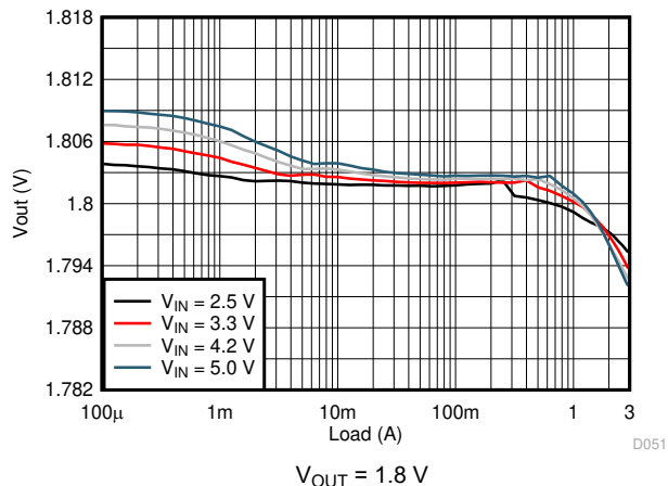
图 8-16. Load Regulation
