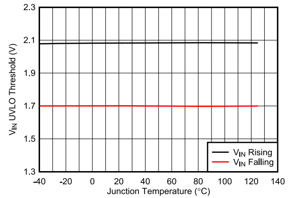
图 6-16. V_{IN} UVLO 上升/下降阈值与结温间的关系
