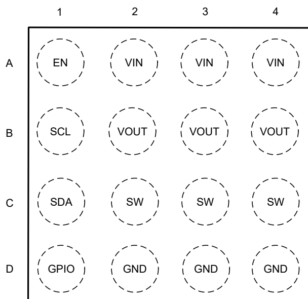
图 5-1. TPS61290x YBG 封装，16 引脚 DSBGA ( 顶视图 )
