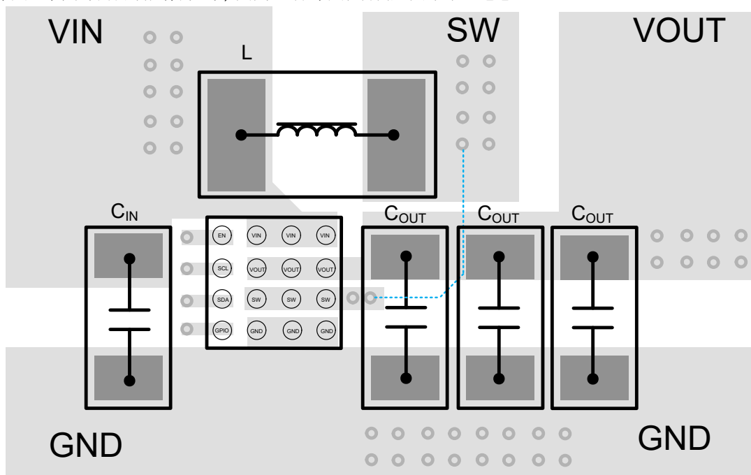
图 9-33. 建议布局 (顶视图)
