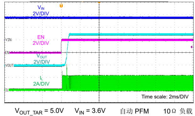
图 9-24. 由 EN 启动
