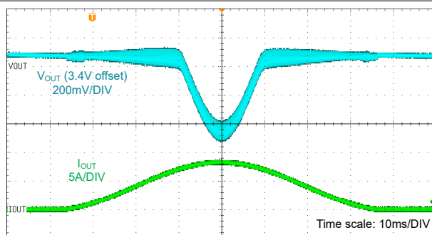
V_{OUT\_TAR} = 3.4V V_{IN} = 2.7V 自动 PFM 负载 = 0A 至 8A 扫描
