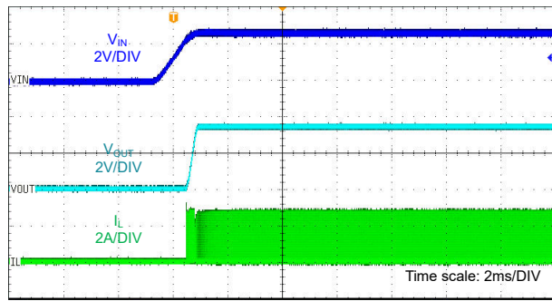
图 9-8. 由 V_{IN} 启动
