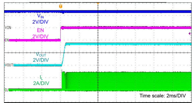
图 9-9. 由 EN 启动
