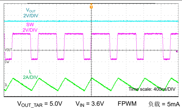
图 9-28. 轻负载条件下的开关波形
