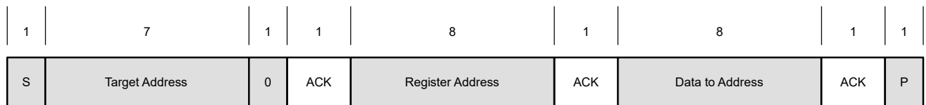
图 7-11. 单字节写入
