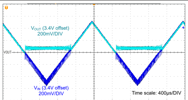
V_{OUT\_TAR} = 3.4V T_A = 25^\circ C 自动 PFM 负载 = 100mA
