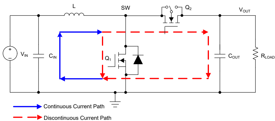
图 9-31. 连续和不连续电流路径
