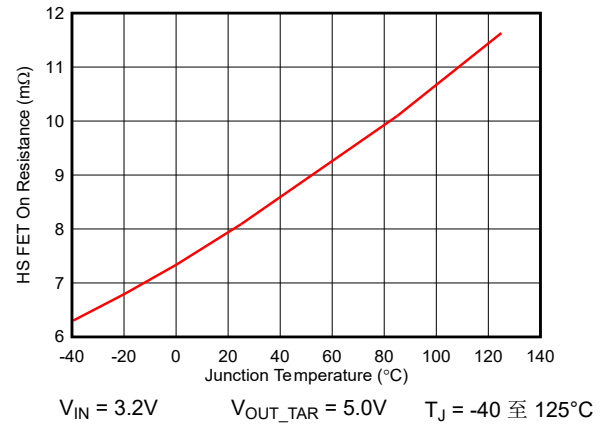
图 6-8. 高侧 R_{ds(on)} 与结温间的关系
