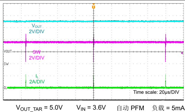
图 9-27. 轻负载条件下的开关波形
