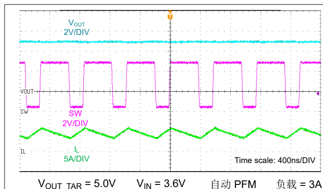
图 9-29. 重负载条件下的开关波形
