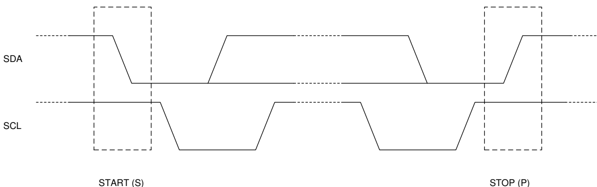
图 7-8. I 2 C START 和 STOP 条件
