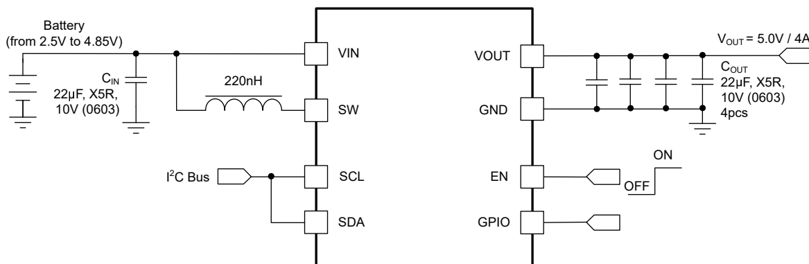
图 9-16. 具有 2.5V - 4.85V V_{IN} 、5.0V V_{OUT} 、4A 输出电流的 TPS61290x
