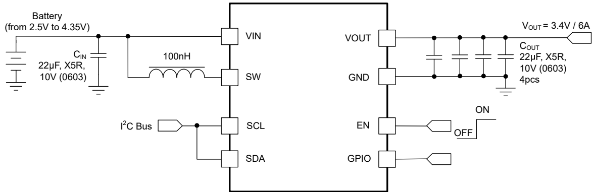
图 9-1. 具有 2.5V – 4.35V V_{IN} 、3.4V V_{OUT} 、6A 输出电流的 TPS61290x
