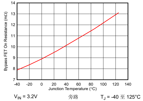
图 6-10. 旁路 FET R_{ds(on)} 与结温间的关系
