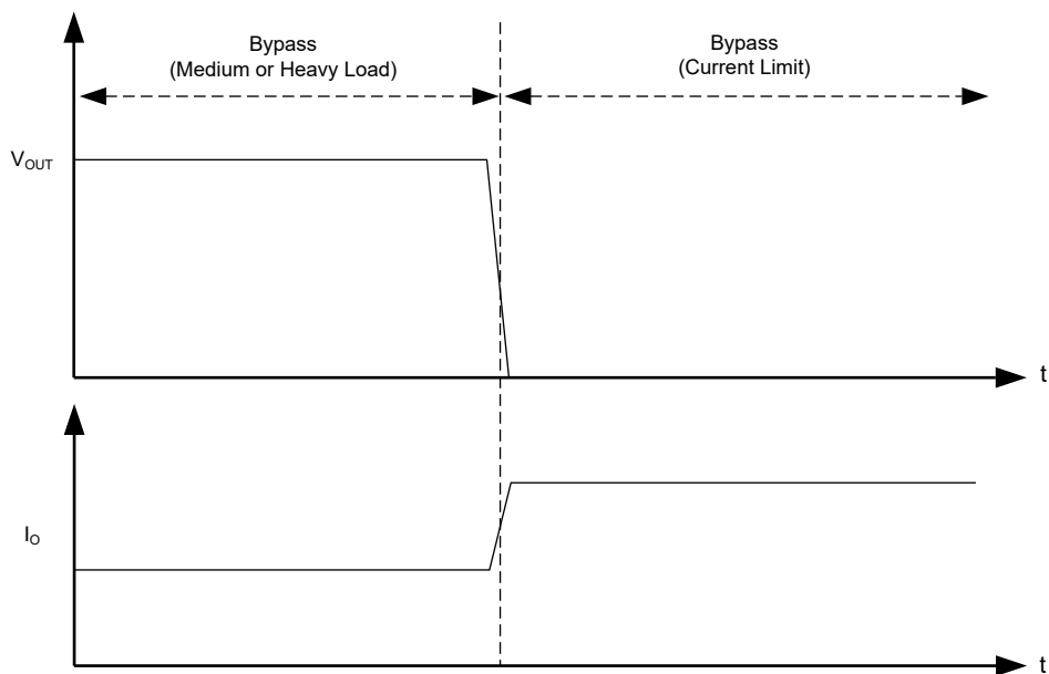
图 7-5. 真旁路模式下的电流限值运行方案
