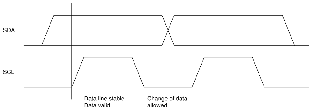
图 7-7. I 2 C 数据有效性
