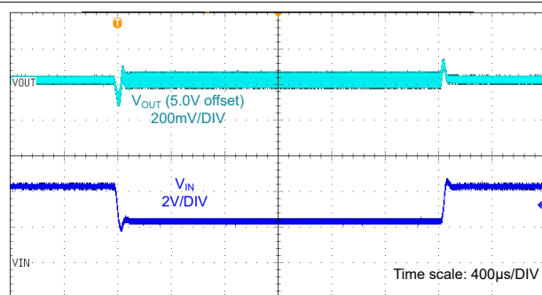
V_{OUT\_TAR} = 5.0V T_A = 25^\circ C 自动 PFM 负载 = 3A V_{IN} = 2.7V 至 4.5V , 20\mu s 压摆率
