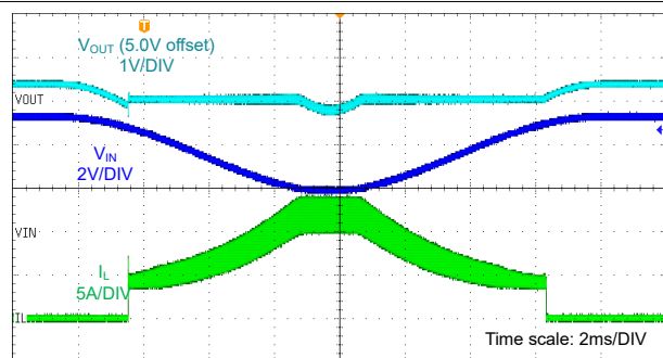
V_{OUT\_TAR} = 5.0V T_A = 25^\circ C 自动 PFM 负载 = 4A V_{IN} = 5.5V 至 2.2V 扫描
