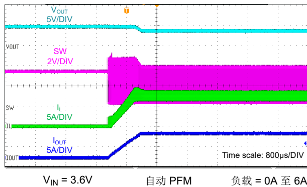
图 9-25. 升压模式下的电流限值运行
