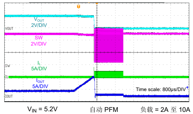
图 9-26. 旁路模式下的电流限值运行
