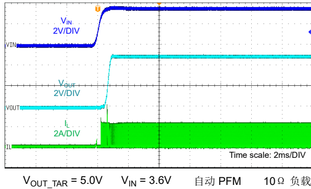
图 9-23. 由 V_{IN} 启动
