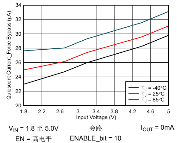
图 6-12. 强制旁路模式下静态电流与输入电压间的关系
