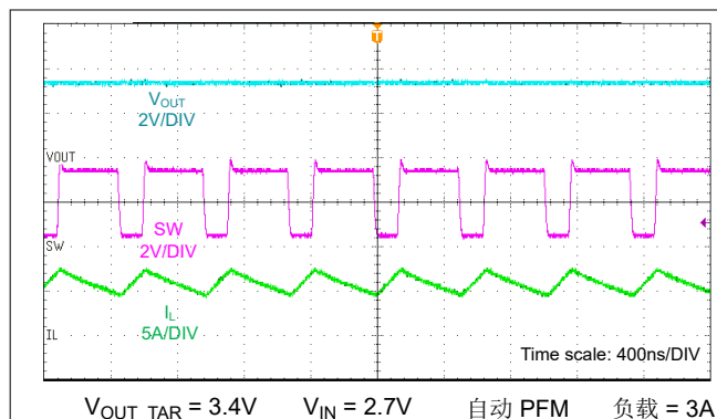
图 9-14. 重负载条件下的开关波形
