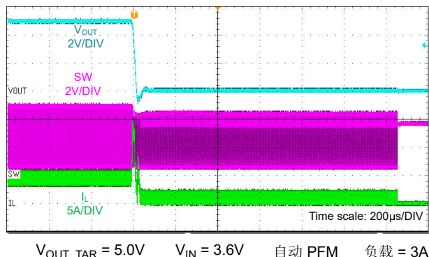
图 9-30. 输出接地短路保护
