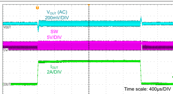
V_{OUT\_TAR} = 3.4V V_{IN} = 2.7V 自动 PFM 负载 = 0.1A - 4A, 0.2A/μs 压摆率
