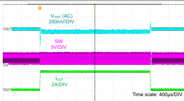
V_{OUT\_TAR} = 5.0V V_{IN} = 3.6V 自动 PFM 负载 = 0.1A - 3A, 0.2A/\mu s 压摆率
