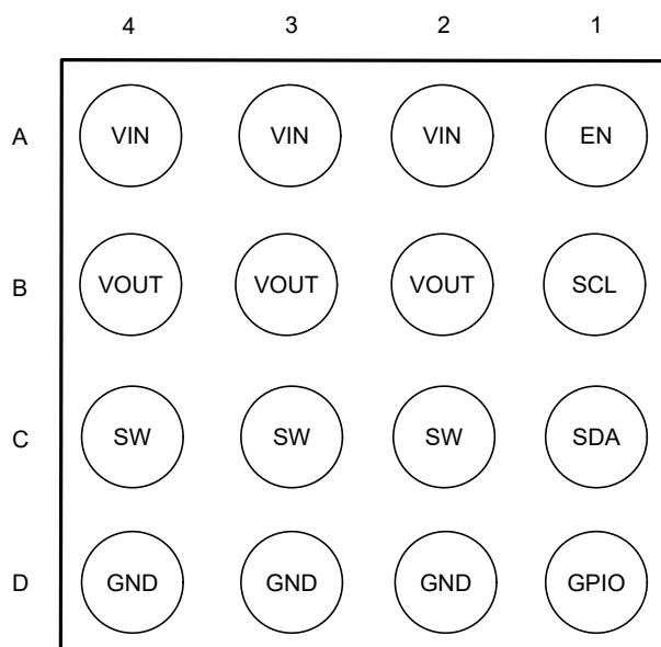
图 5-2. TPS61290x YBG 封装，16 引脚 DSBGA ( 底视图 )
