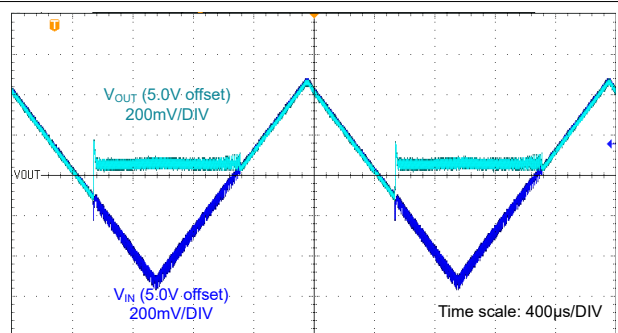
V_{OUT\_TAR} = 5.0V T_A = 25^\circ C 自动 PFM 负载 = 100mA
