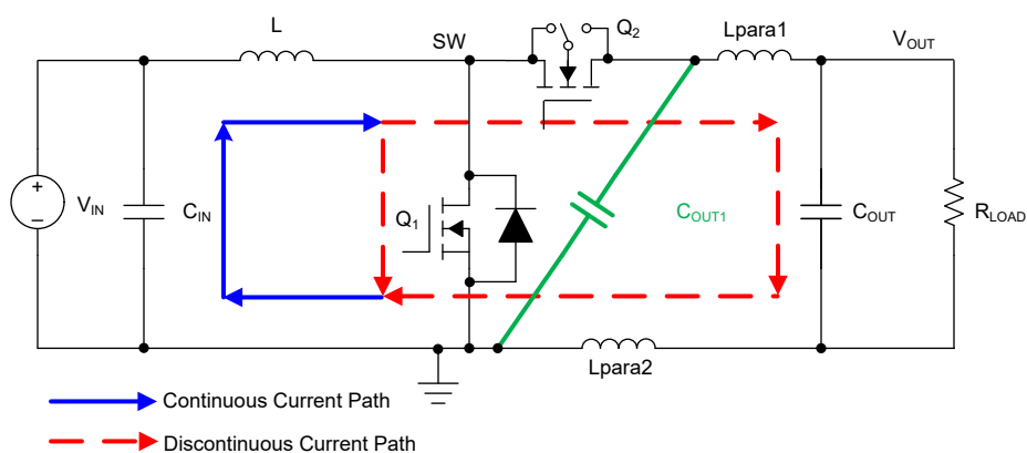
图 9-32. 不连续电流路径中的 PCB 寄生电感器
