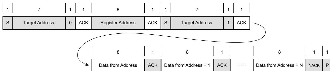
图 7-14. 多字节读取
