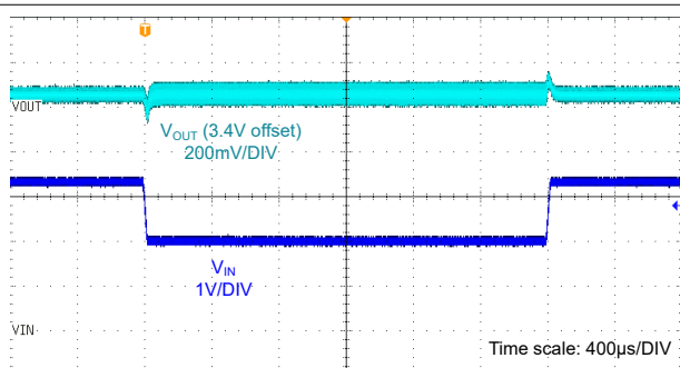
V_{OUT\_TAR} = 3.4V T_A = 25^\circ C 自动 PFM 负载 = 4A V_{IN} = 2V 至 3.4V , 20μs 压摆率
