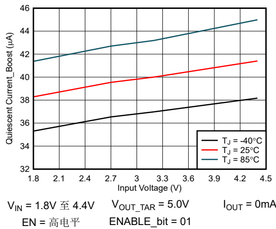
图 6-11. 升压模式下静态电流与输入电压间的关系
