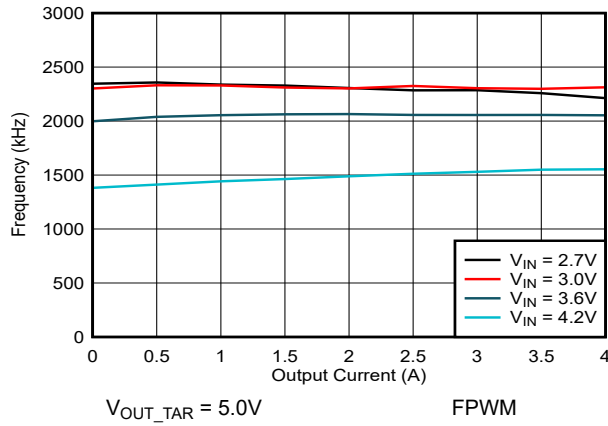
图 6-7. 开关频率与输出电流间的关系
