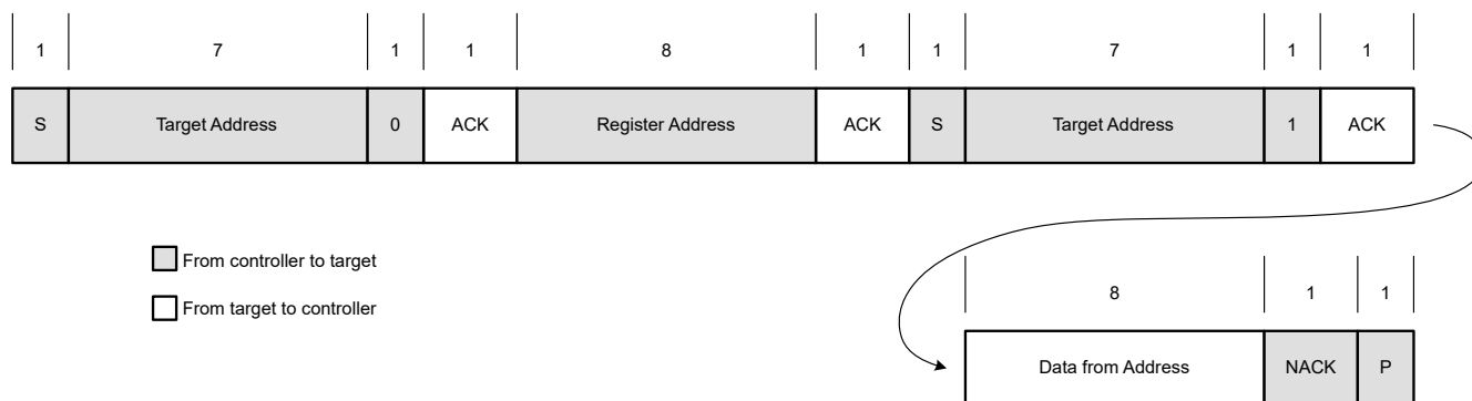
图 7-12. 单字节读取
