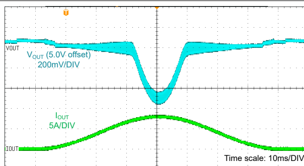
V_{OUT\_TAR} = 5.0V V_{IN} = 3.6V 自动 PFM 负载 = 0A 至 6A 扫描
