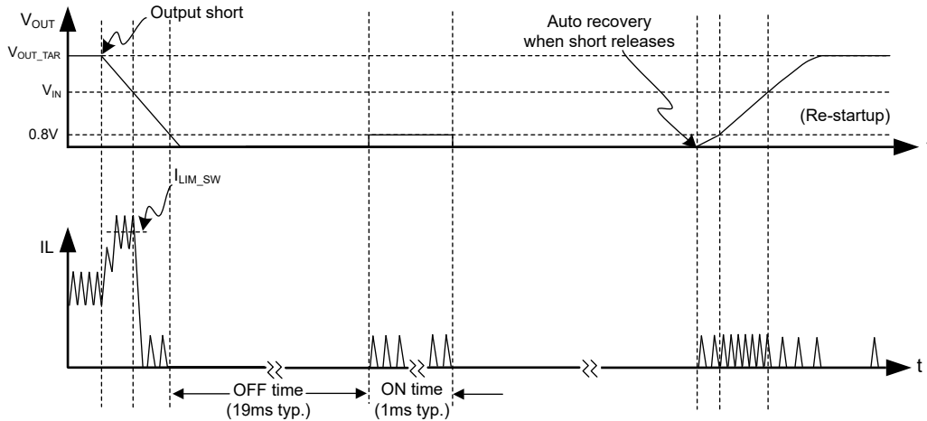
图 7-6. OSGP 的断续模式
