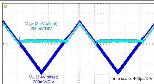
V_{OUT\_TAR} = 3.4V T_A = 25^\circ C 自动 PFM 负载 = 4A
