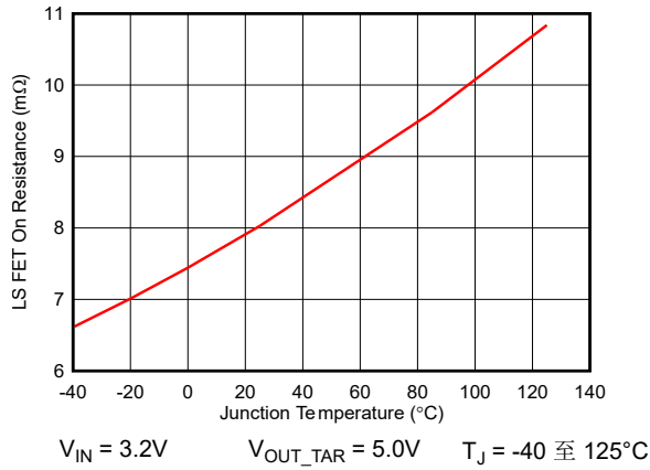
图 6-9. 低侧 R_{ds(on)} 与结温间的关系
