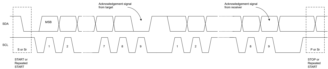
图 7-9. 字节格式
