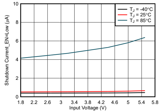
图 6-14. EN = 低电平时关断电流与输入电压间的关系
