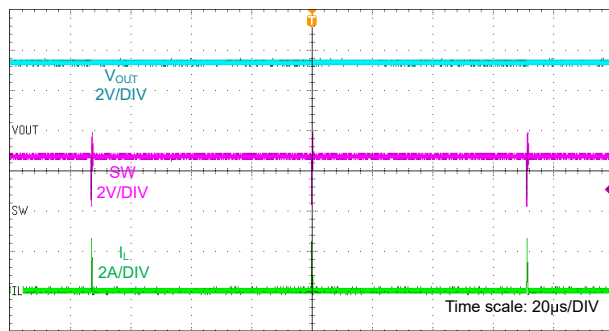
图 9-10. 升压模式下的电流限值运行
