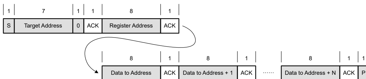
图 7-13. 多字节写入
