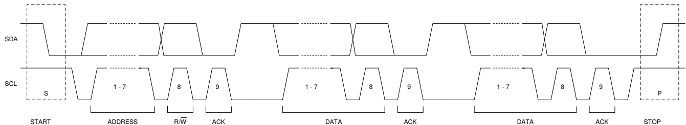
图 7-10. 目标地址和数据方向
