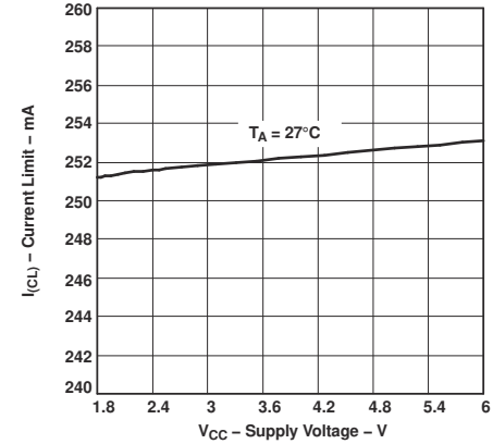
图 5-8. TPS61041 电流量值与电源电压之间的关系
