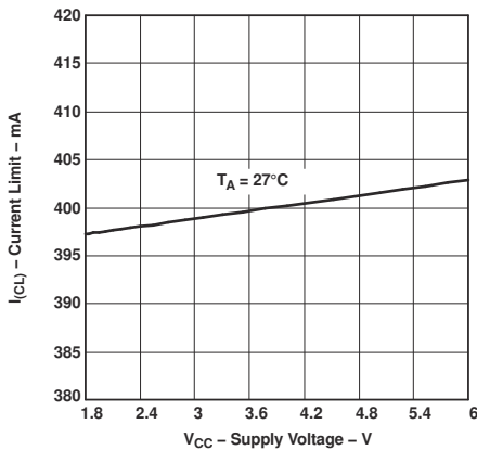
图 5-9. TPS61040 电流量值与电源电压之间的关系
