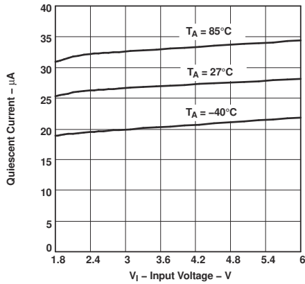
图 5-5. TPS61040 静态电流与输入电压之间的关系
