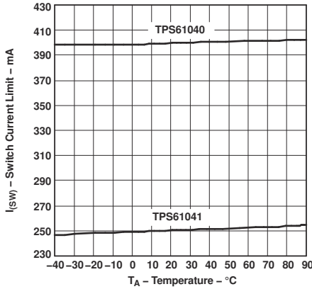
图 5-7. TPS6104x 开关电流量值与自然通风条件下的温度之间的关系
