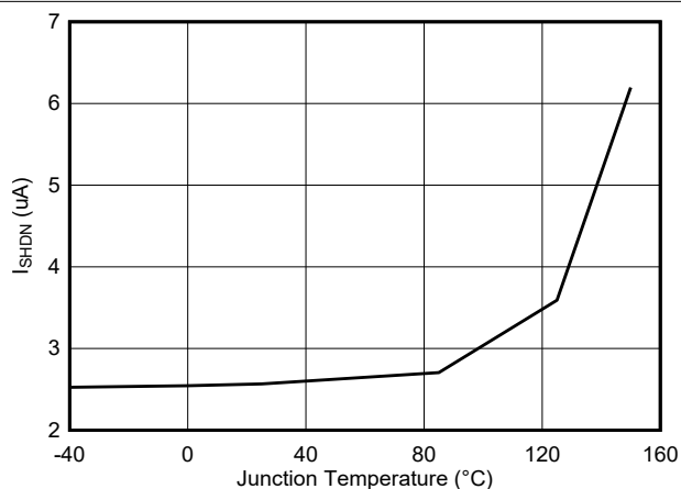
图 5-2. 关断电流与温度间的关系
