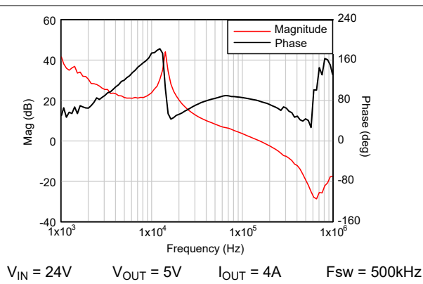
图 7-5. 波特图
