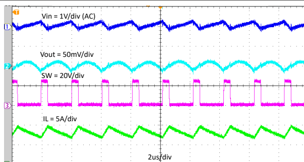
图 7-9. 稳态波形, I_{OUT} = 8A
