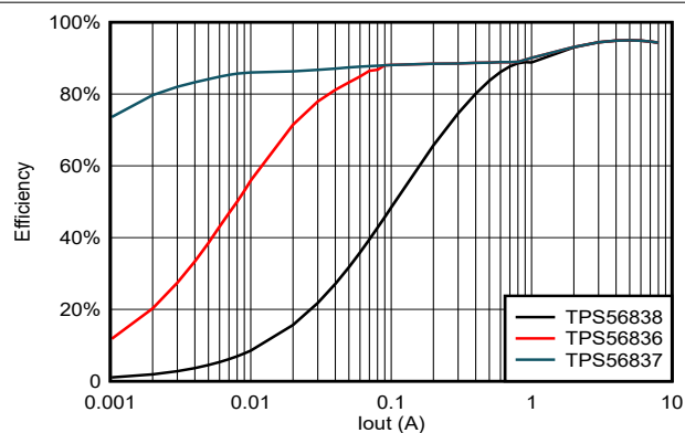
图 5-22. TPS56837、TPS56838 和 TPS56836 效率, V_{in} = 24V , V_{out} = 5V , F_{sw} = 500kHz
