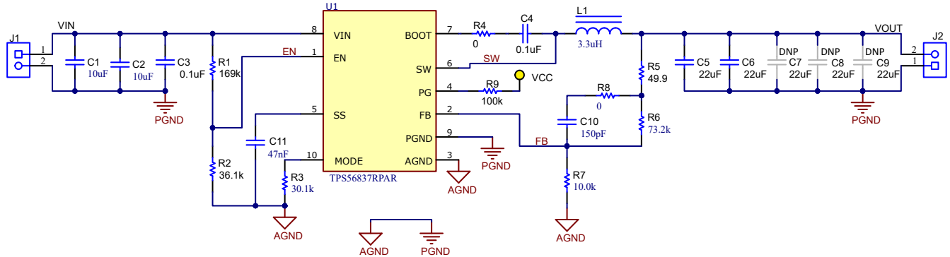
图 7-1. TPS56837 5V、8A 参考设计
