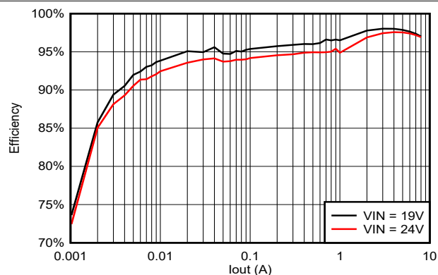
图 5-20. TPS56837 效率, V_{out} = 12V , F_{sw} = 500kHz
