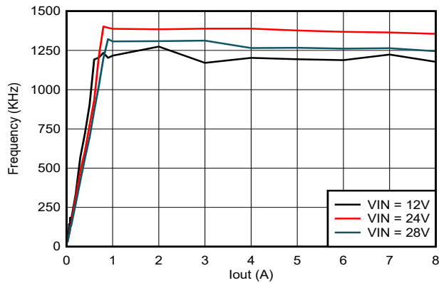
图 5-15. TPS56837 开关频率与输出电流间的关系, V_{out} = 5V , F_{sw} = 1200kHz
