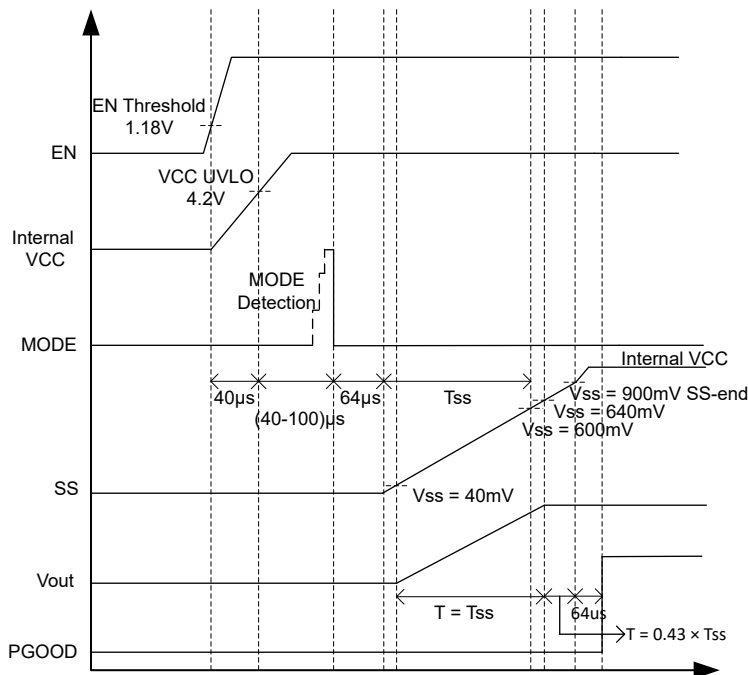
图 6-1. 上电序列
