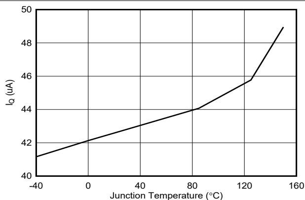
图 5-1. TPS56837 静态电流与温度间的关系
