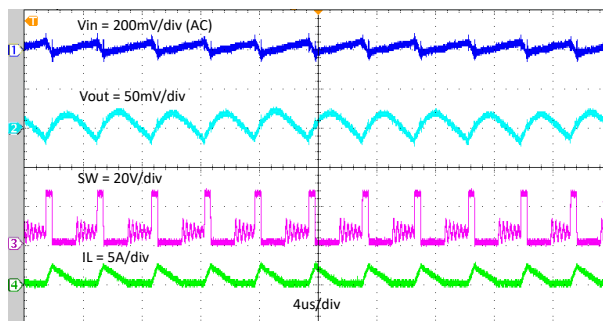
图 7-7. 稳态波形, I_{OUT} = 0.6A
