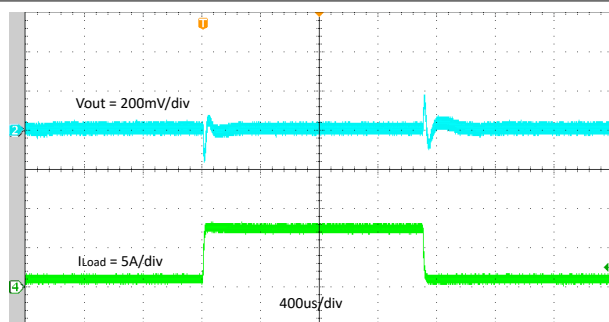
图 7-12. 瞬态响应 (0.8A 到 7.2A)
