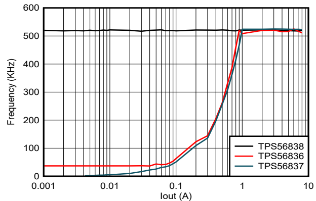
图 5-16. TPS56837、TPS56838 和 TPS56836 开关频率与输出电流间的关系, V_{in} = 24V , V_{out} = 5V , F_{sw} = 500kHz
