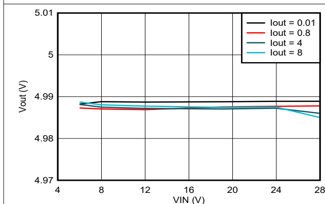
图 7-4. 线性调整率
