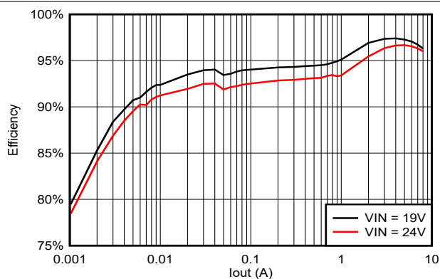
图 5-21. TPS56837 效率, V_{out} = 12V , F_{sw} = 800kHz
