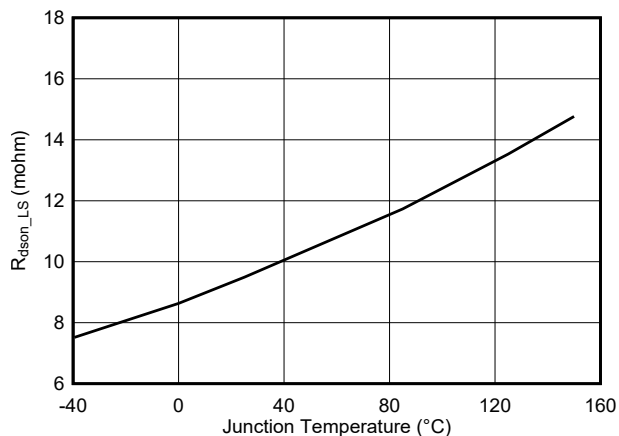
图 5-4. 低侧 R_{DS(on)} 与温度间的关系
