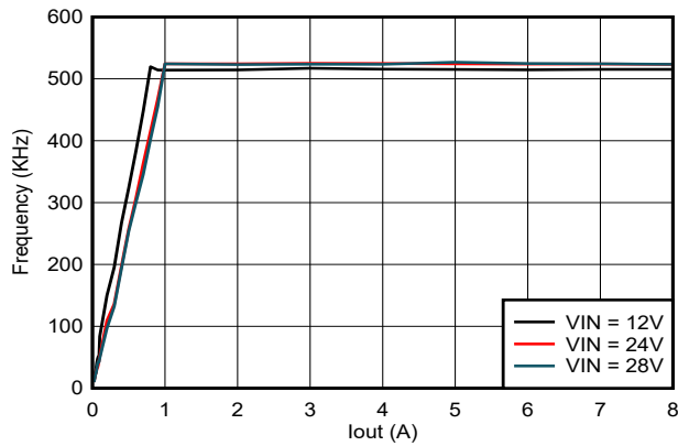
图 5-13. TPS56837 开关频率与输出电流间的关系, V_{out} = 5V , F_{sw} = 500kHz
