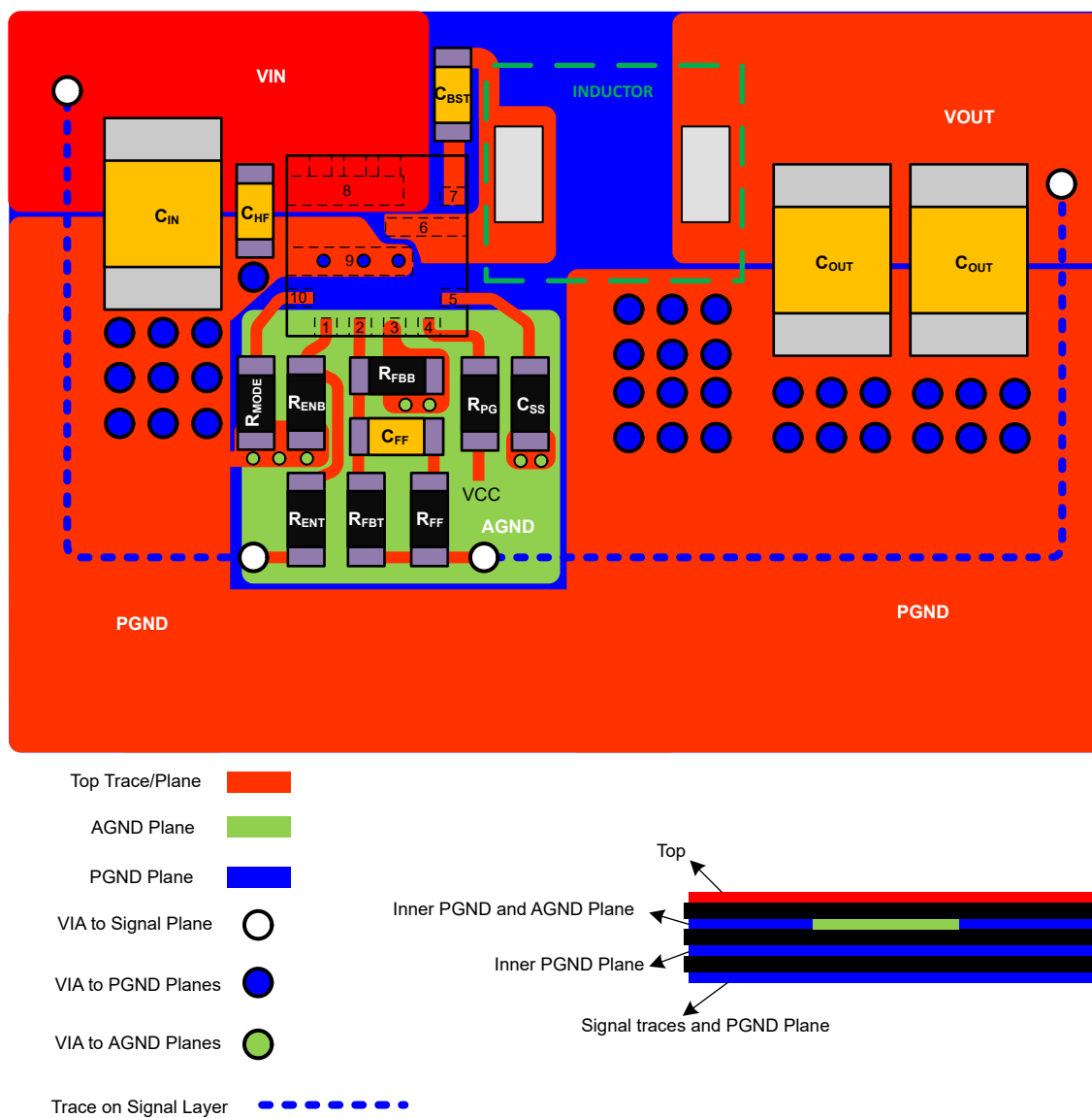
图 7-18. TPS56837 布局
