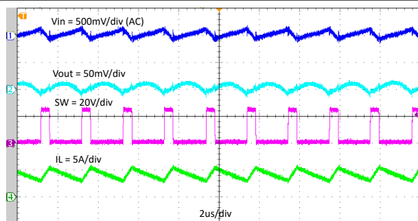
图 7-8. 稳态波形, I_{OUT} = 4A
