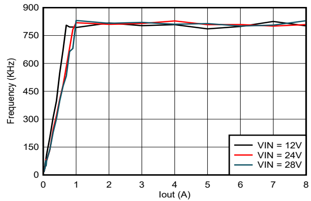
图 5-14. TPS56837 开关频率与输出电流间的关系, V_{out} = 5V , F_{sw} = 800kHz
