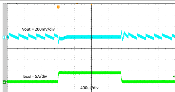
图 7-10. 瞬态响应 (0A 到 4A)
