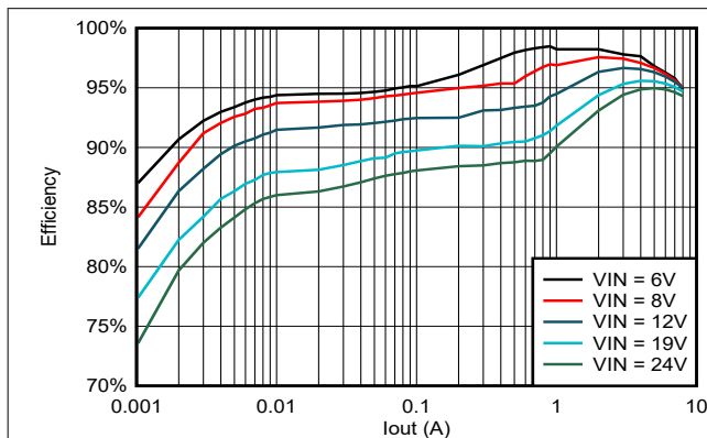
图 7-2. 效率
