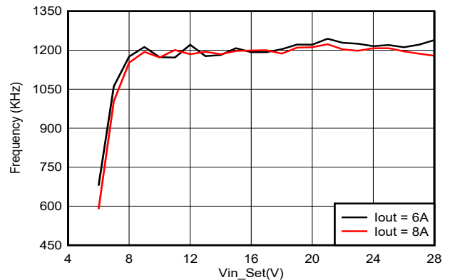
图 5-12. 开关频率与输入电压间的关系, V_{out} = 5V , F_{sw} = 1200kHz
