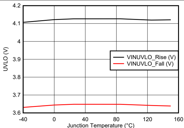
图 5-6. VIN UVLO 与温度间的关系
