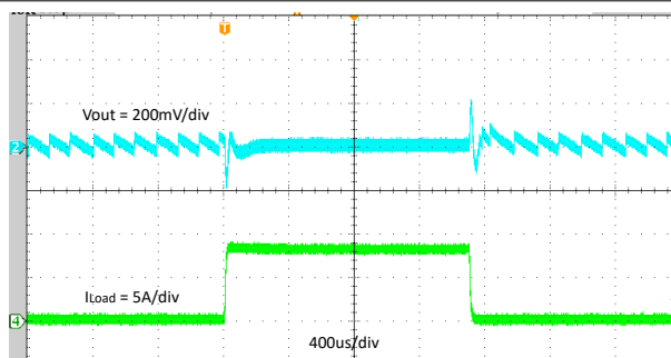
图 7-11. 瞬态响应 (0A 到 8A)
