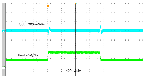
图 7-13. 瞬态响应 (4A 到 8A)
