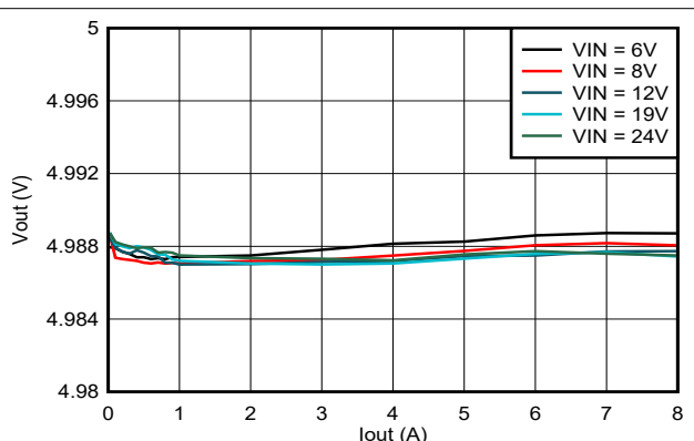
图 7-3. 负载调整率
