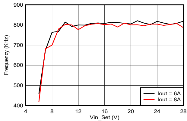
图 5-11. 开关频率与输入电压间的关系, V_{out} = 5V , F_{sw} = 800kHz
