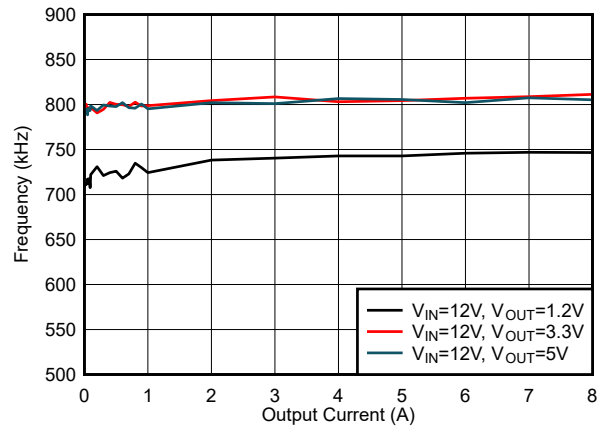
图 6-32. f_{SW} 负载调节, 模式 = FCCM, f_{SW} = 800kHz
