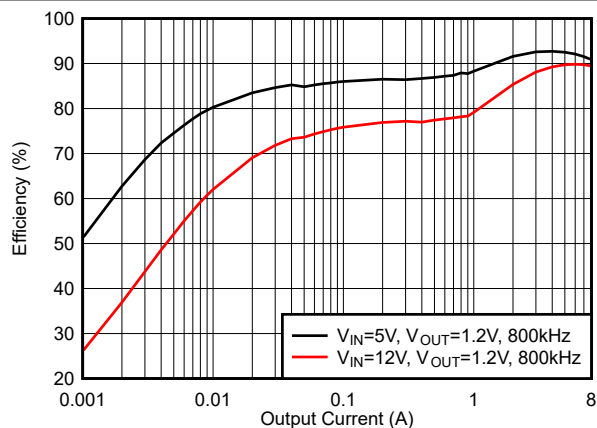
图 6-13. 效率, 模式 = DCM, f_{SW} = 800kHz
