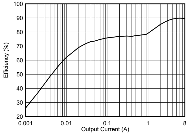
图 8-2. 效率
