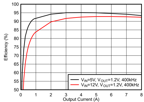
图 6-12. 效率, 模式 = FCCM, f_{SW} = 400kHz
