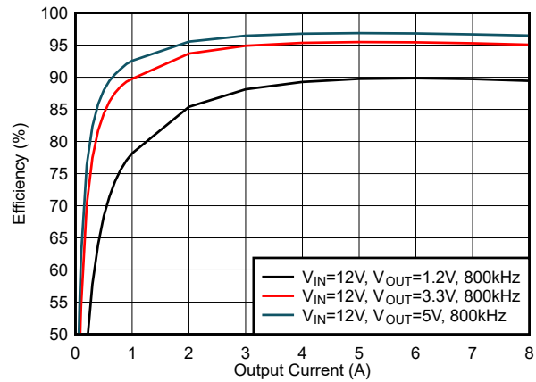
图 6-20. 效率, 模式 = FCCM, f_{SW} = 800kHz
