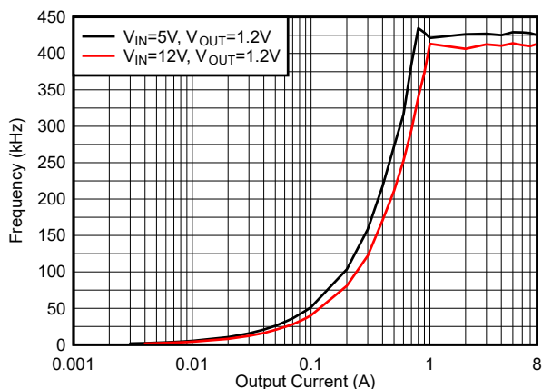
图 6-25. f_{SW} 负载调节, 模式 = DCM, f_{SW} = 400kHz
