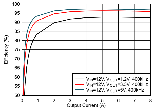
效率，FCCM 模式
