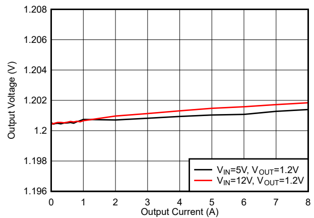
图 6-24. 负载调节, f_{SW} = 800kHz
