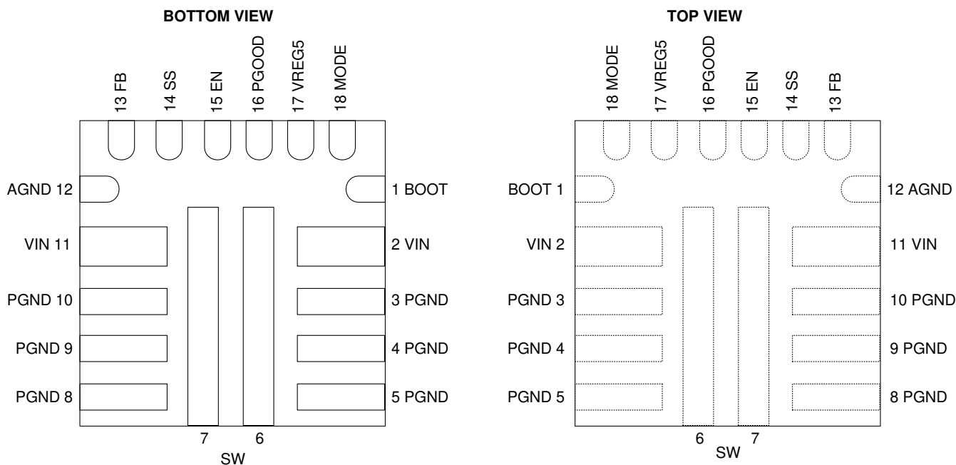
图 5-1. 18 引脚 VQFN RNN 封装（左底视图、右顶视图）
