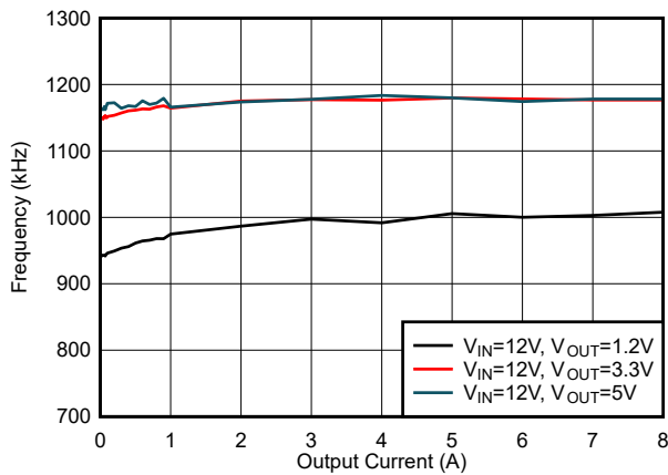
图 6-33. f_{SW} 负载调节, 模式 = FCCM, f_{SW} = 1200kHz
