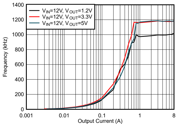
图 6-36. f_{SW} 负载调节, 模式 = DCM, f_{SW} = 1200kHz
