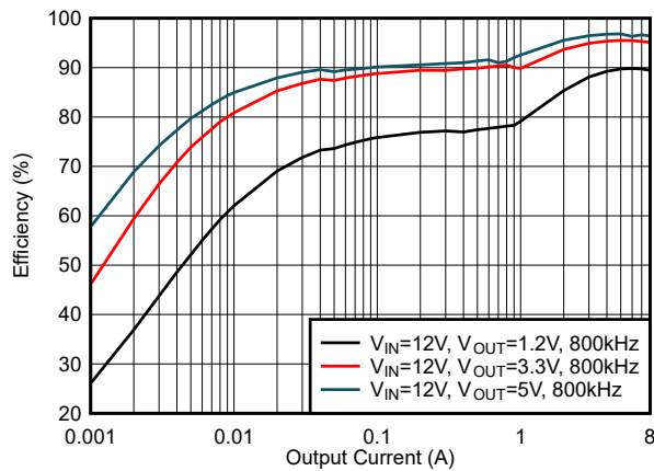
图 6-19. 效率, 模式 = DCM, f_{SW} = 800kHz
