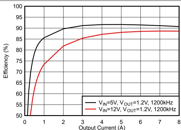
图 6-16. 效率, 模式 = FCCM, f_{SW} = 1200kHz
