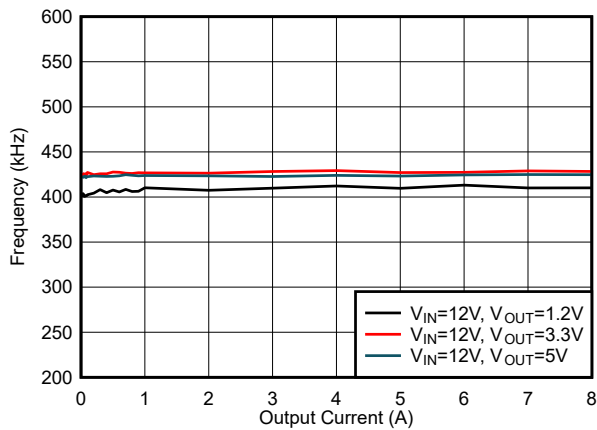
图 6-31. f_{SW} 负载调节, 模式 = FCCM, f_{SW} = 400kHz
