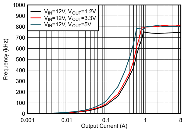
图 6-35. f_{SW} 负载调节, 模式 = DCM, f_{SW} = 800kHz
