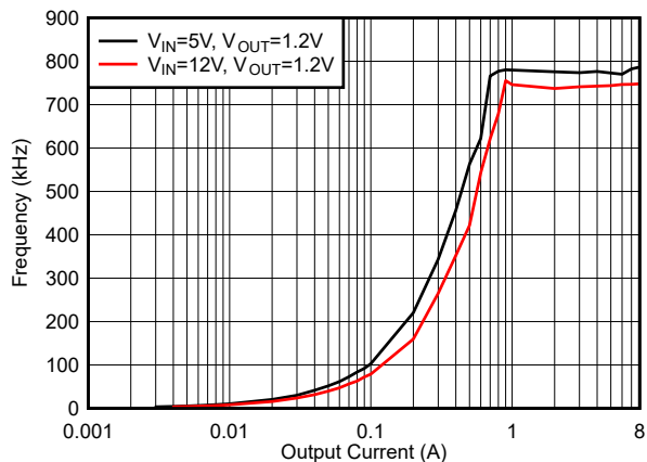
图 6-26. f_{SW} 负载调节, 模式 = DCM, f_{SW} = 800kHz
