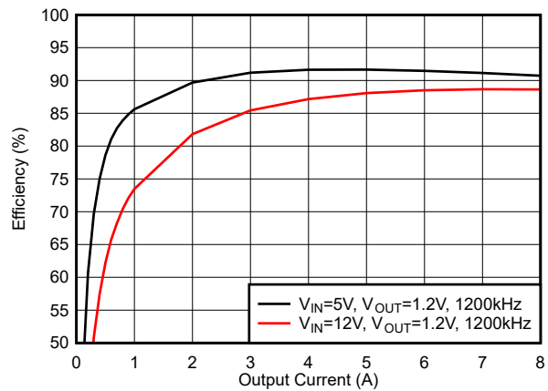
图 6-22. 效率, 模式 = FCCM, f_{SW} = 1200kHz
