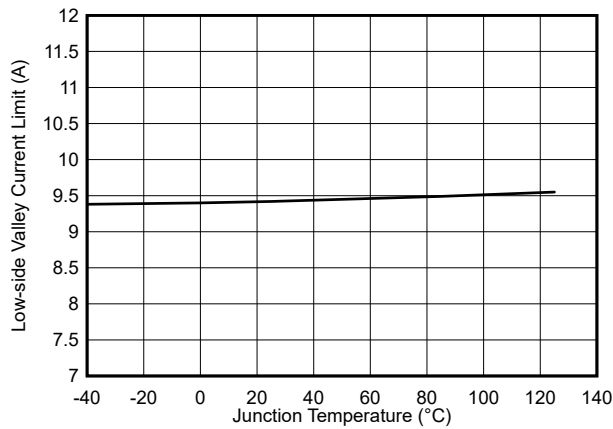
图 6-9. TPS568231 电流限制 (ILIM) 与温度间的关系
