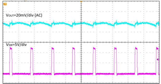
图 8-5. 输出电压纹波, I_{OUT} = 8A , 时间 = 1 \mu S/div
