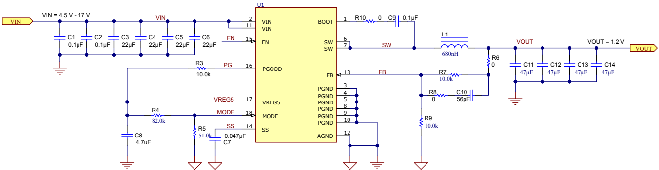
图 8-1. 应用原理图
