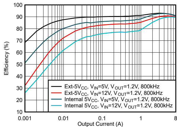
图 6-23. 效率, 外部 VCC 与内部 VCC, 模式 = DCM, f_{SW} = 800kHz
