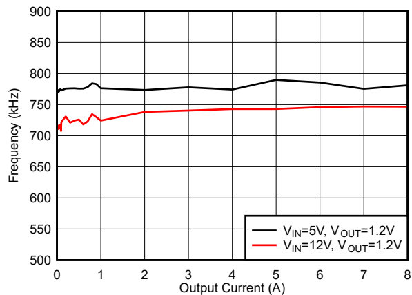
图 6-29. f_{SW} 负载调节, 模式 = FCCM, f_{SW} = 800kHz
