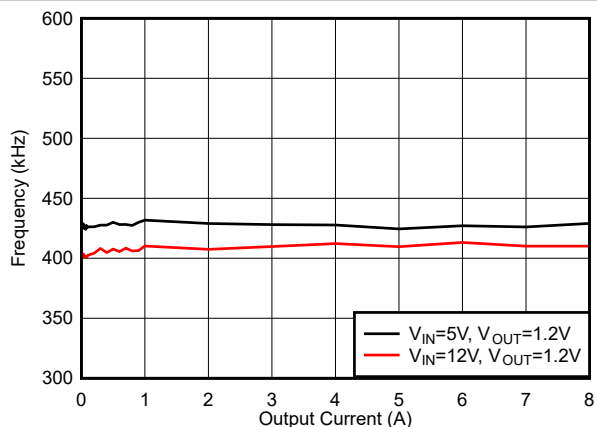
图 6-28. f_{SW} 负载调节, 模式 = FCCM, f_{SW} = 400kHz
