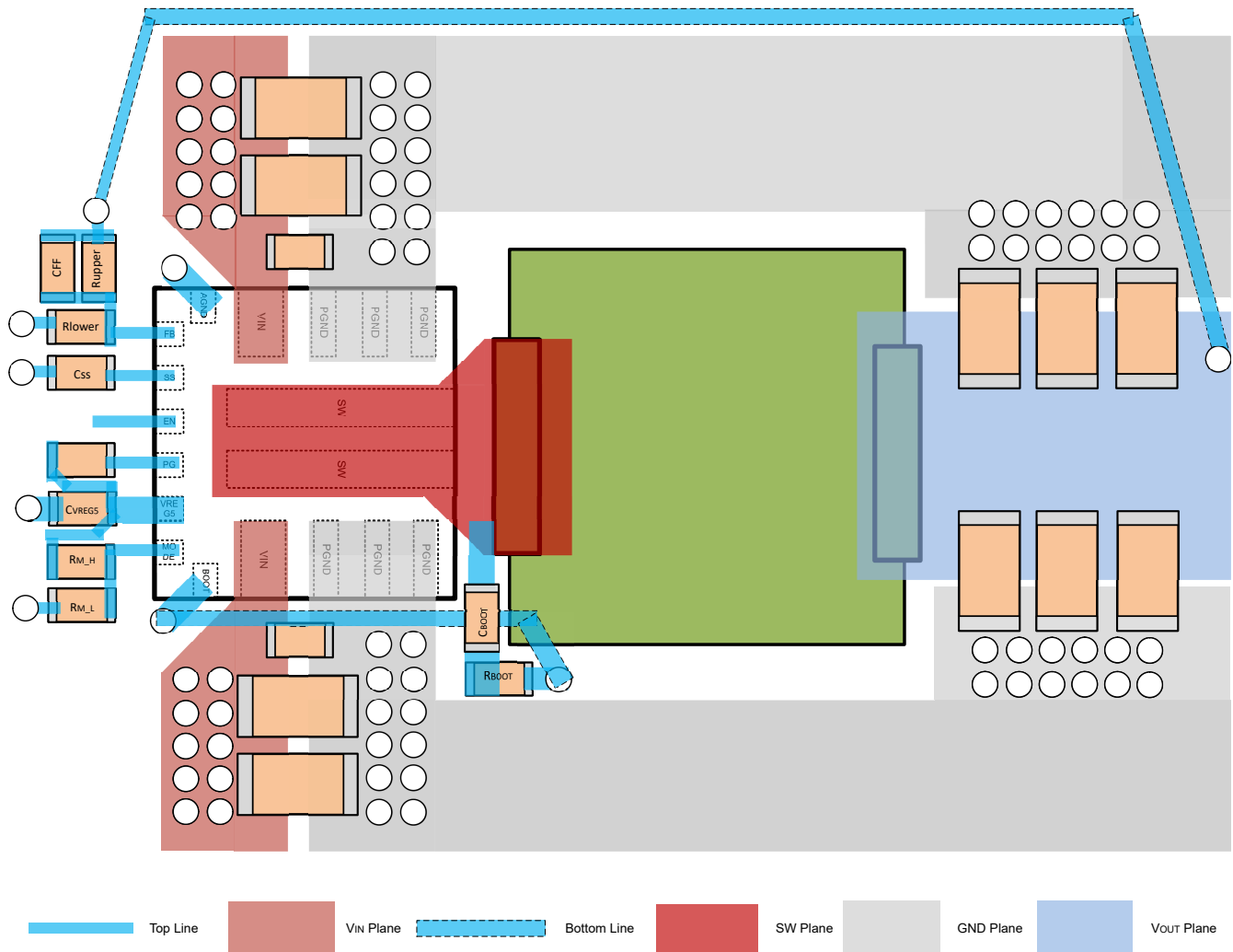
图 8-8. 布局示例
