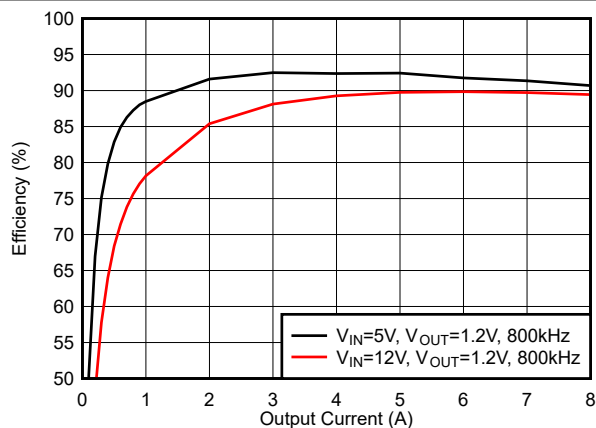
图 6-14. 效率, 模式 = FCCM, f_{SW} = 800kHz
