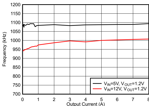
图 6-30. f_{SW} 负载调节, 模式 = FCCM, f_{SW} = 1200kHz
