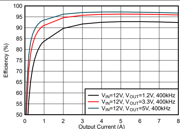
图 6-18. 效率, 模式 = FCCM, f_{SW} = 400kHz
