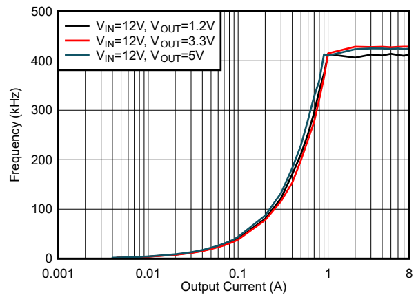
图 6-34. f_{SW} 负载调节, 模式 = DCM, f_{SW} = 400kHz
