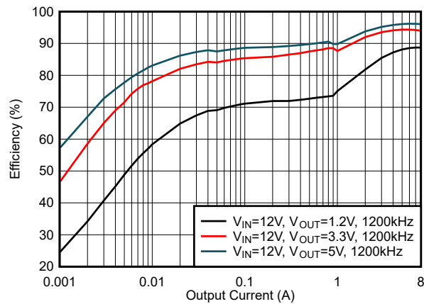
图 6-21. 效率, 模式 = DCM, f_{SW} = 1200kHz
