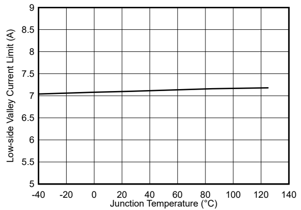
图 6-10. TPS568231 电流限制 (ILIM-1) 与温度间的关系
