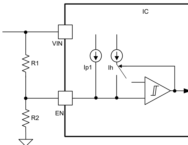
图 7-2. 可调节 V_{IN} 欠压锁定
