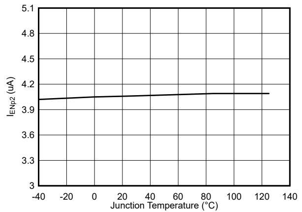
图 6-8. 使能上拉电流, V_{EN} = 1.3V
