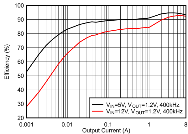
图 6-11. 效率, 模式 = DCM, f_{SW} = 400kHz
