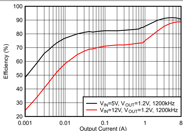
图 6-15. 效率, 模式 = DCM, f_{SW} = 1200kHz
