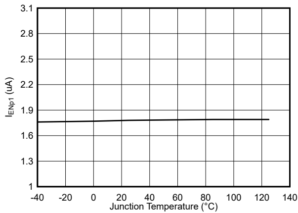
图 6-7. 使能上拉电流, V_{EN} = 1V
