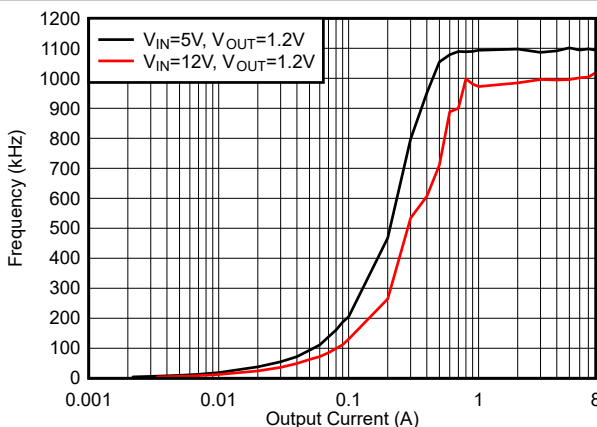
图 6-27. f_{SW} 负载调节, 模式 = DCM, f_{SW} = 1200kHz
