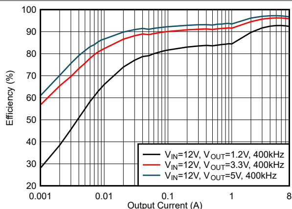
图 6-17. 效率, 模式 = DCM, f_{SW} = 400kHz
