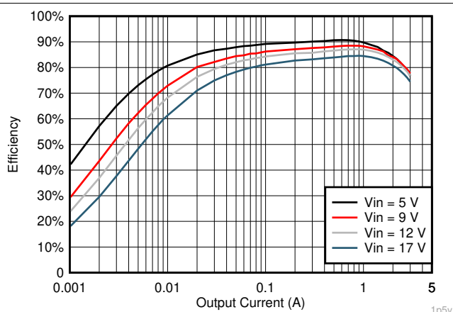
图 6-11. V_{OUT} = 1.5V 效率, L = 1.5\mu H
