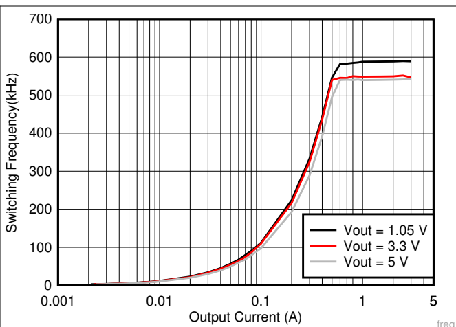
图 6-8. 开关频率与输出电流间的关系
