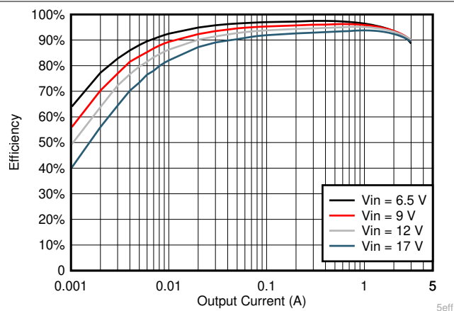
图 6-14. V_{OUT} = 5V 效率, L = 4.7\mu H
