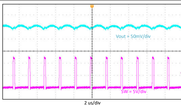
图 8-7. 输出电压纹波, I_{out} = 3A
