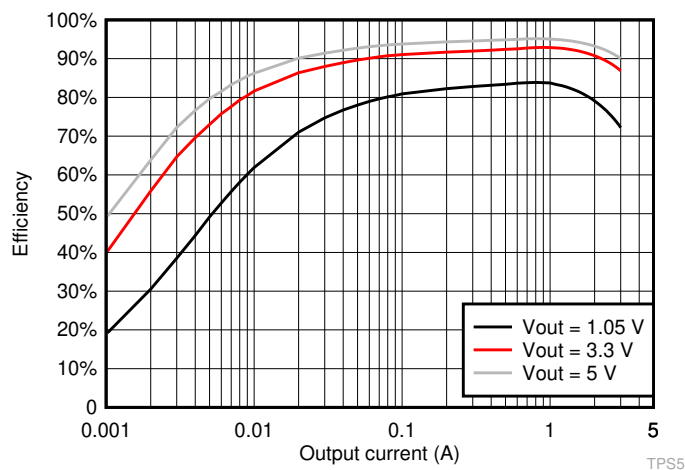
TPS563202 效率
