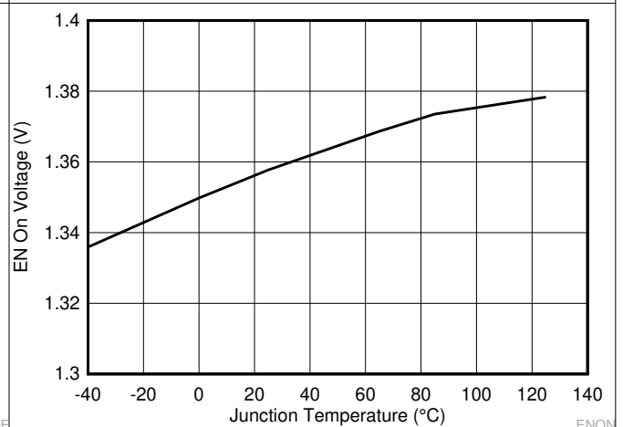
图 6-4. EN 引脚 EN 导通电压与结温间的关系
