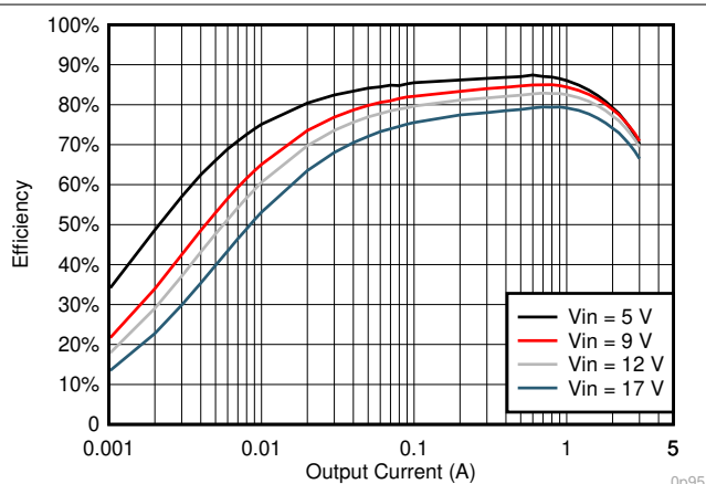
图 6-9. V_{OUT} = 0.95V 效率, L = 1.2\mu H
