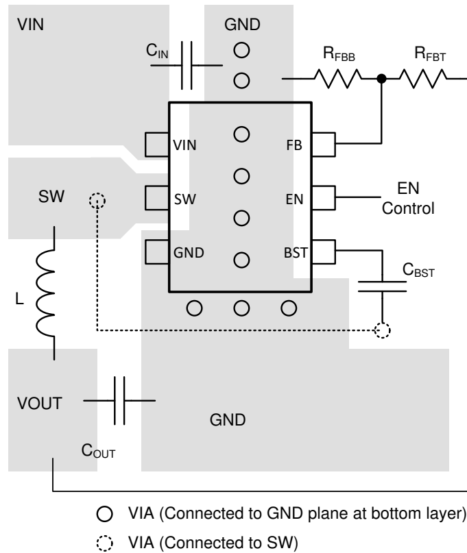
图 9-1. TPS563202 布局
