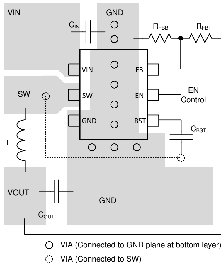
图 22. TPS562231 Layout
