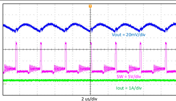
图 9-6. 输出电压纹波, I_{out} = 0.2A
