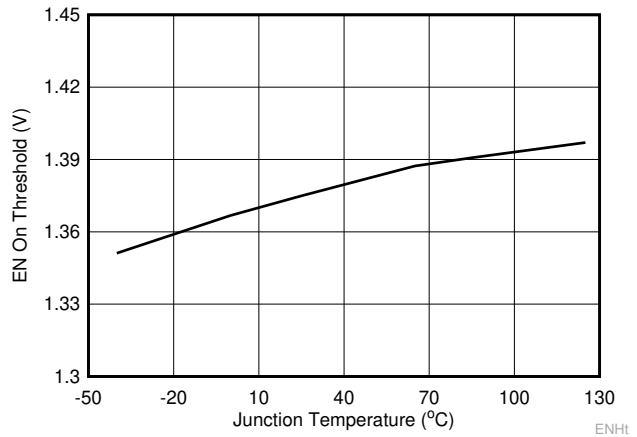
图 7-4. EN 导通阈值电压与结温间的关系
