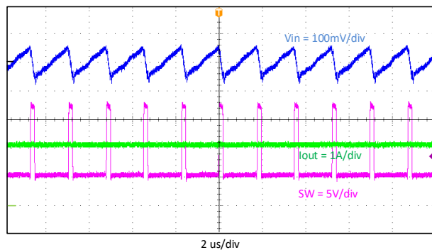
图 9-4. 输入电压纹波 I_{out} = 2A
