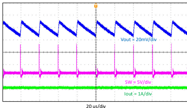
图 9-5. 输出电压纹波, I_{out} = 0.01A
