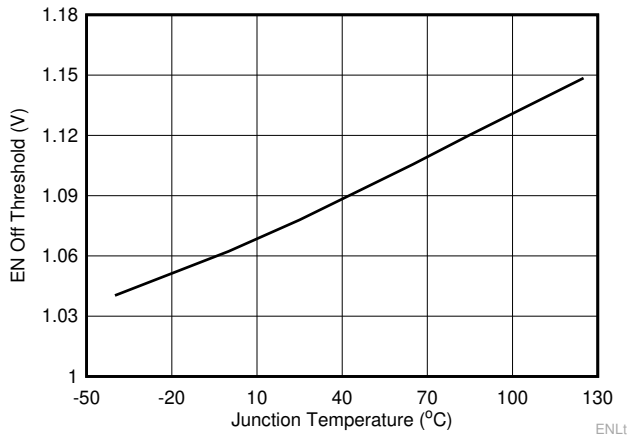
图 7-3. EN 关断阈值电压与结温间的关系
