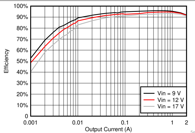
图 7-14. V_{OUT} = 5V 效率, L = 4.7\mu H
