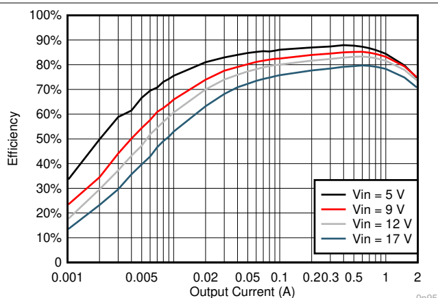
图 7-9. V_{OUT} = 0.95V 效率, L = 2.2\mu H
