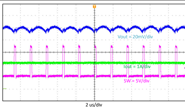
图 9-7. 输出电压纹波, I_{out} = 2A
