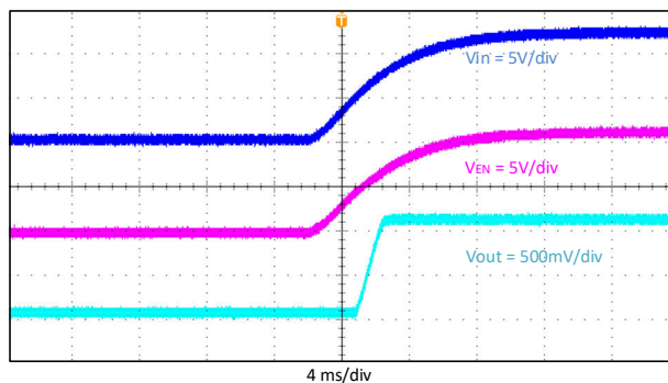
图 9-8. 相对于 VIN 的启动
