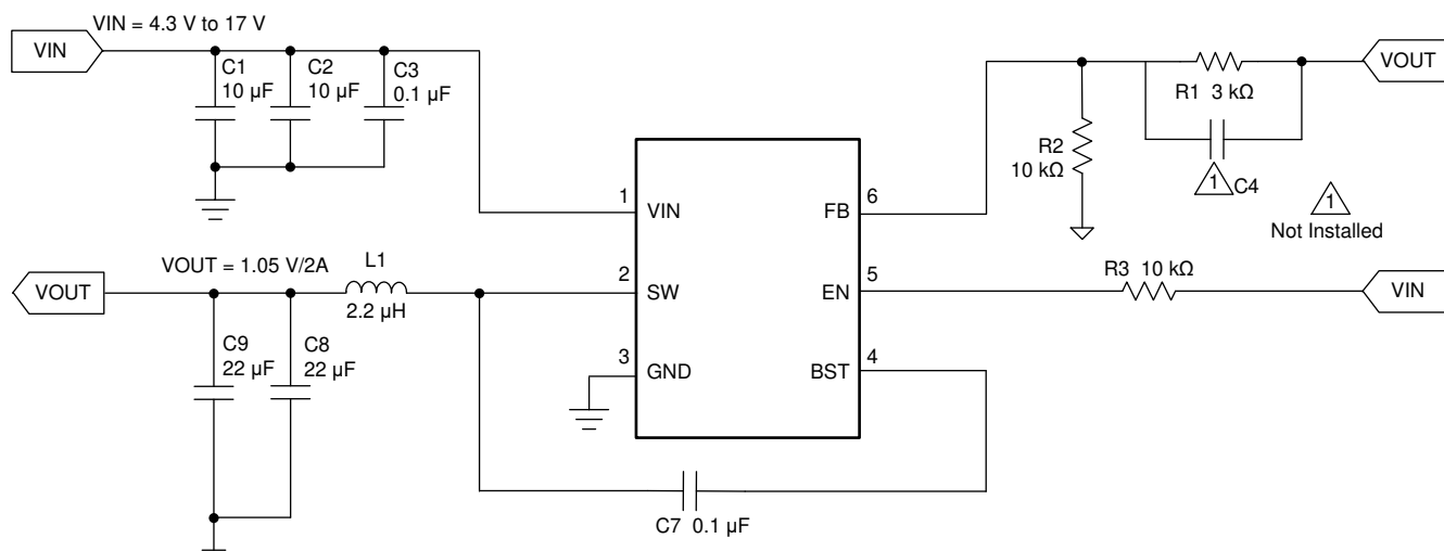
图 9-1. 1.05V、2A 参考设计
