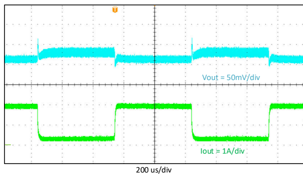
图 9-12. 瞬态响应, 0.2A 到 1.8A
