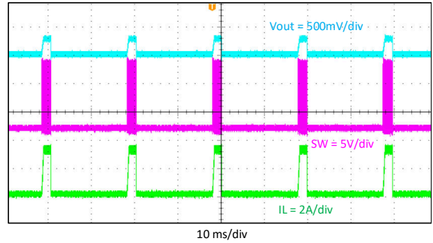
图 9-15. 断续, I_{out} = 5A
