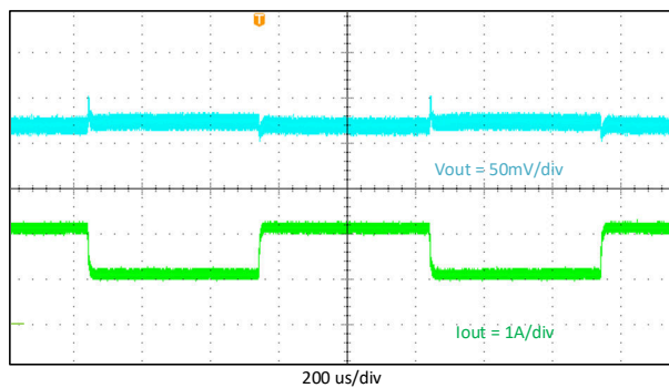
图 9-13. 瞬态响应, 1A 到 2A
