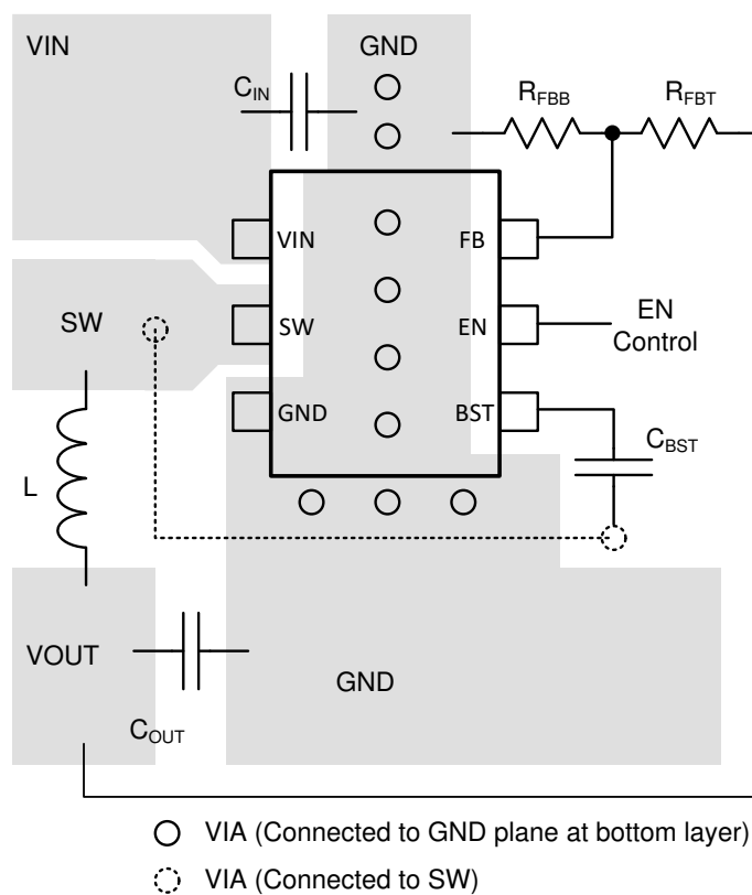
图 11-1. TPS562202 布局
