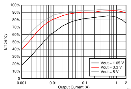
TPS562202 效率
