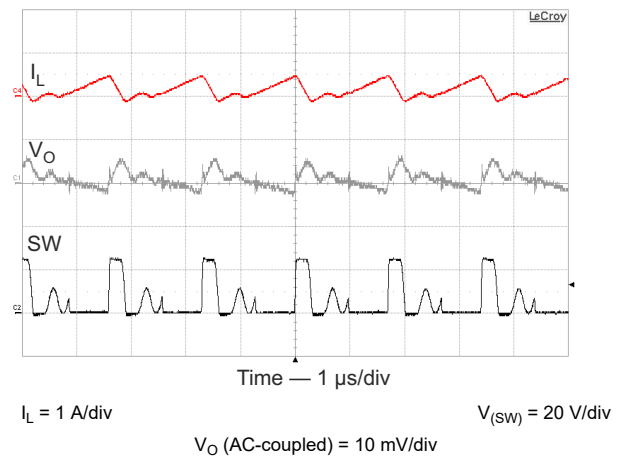
图 8-6. DCM PWM Operation
