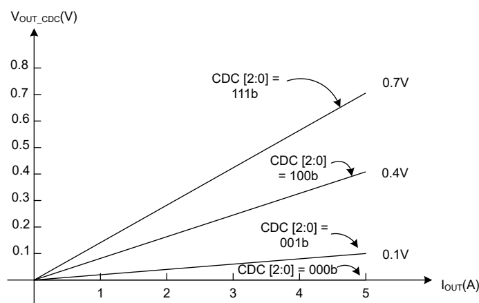
图 6-5. 输出电压上升值与输出电流间的关系
