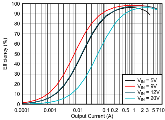
图 5-3. 效率与输出电流间的关系, V_{OUT} = 9V , FPWM
