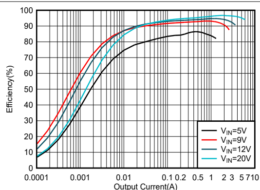
图 5-10. 效率与输出电流间的关系, V_{OUT} = 20V , PFM
