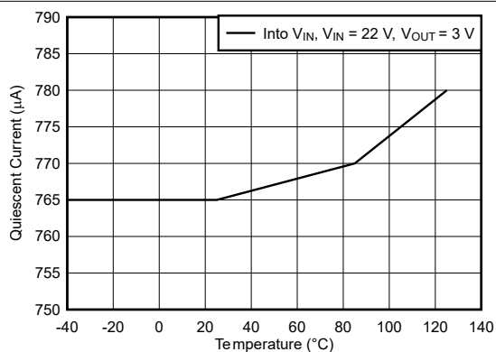
图 5-13. 静态电流与温度间的关系
