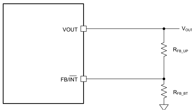
图 6-4. 由外部电阻分压器设置输出电压
