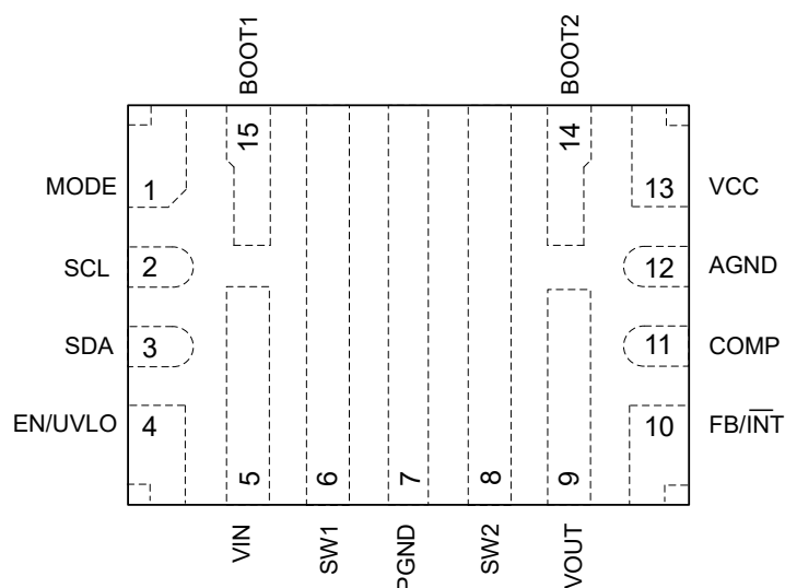
图 4-1. TPS55285A VAL 封装，15 引脚 WQFN-HR (透明顶视图)
