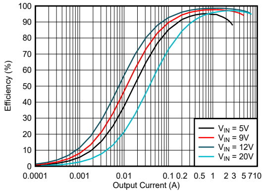
图 5-5. 效率与输出电流间的关系, V_{OUT} = 12V , FPWM
