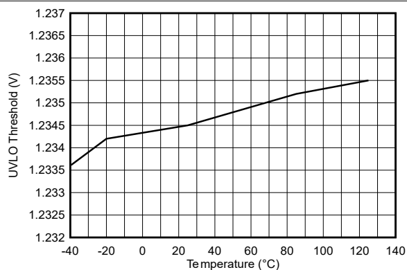
图 5-14. ENABLE/UVLO 上升阈值与温度间的关系
