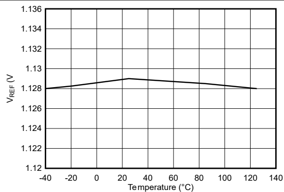
图 5-12. 基准电压与温度间的关系 ( V_{REF} = 1.129V )
