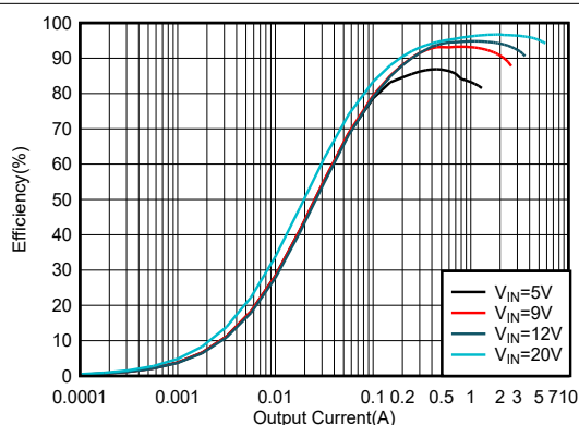
图 5-9. 效率与输出电流间的关系, V_{OUT} = 20V , FPWM
