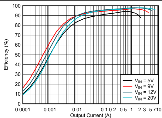
图 5-8. 效率与输出电流间的关系, V_{OUT} = 15V , PFM
