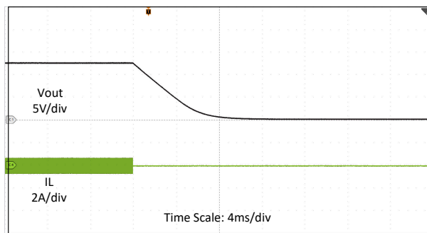
图 8-15. V_{IN} = 12V 、 V_{OUT} = 5V 、 I_{OUT} = 0A 时的输出放电
