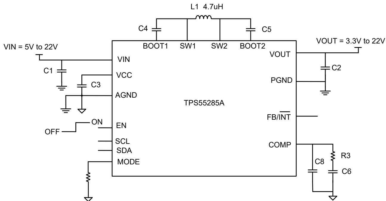
图 8-1. 输入电压为 5V 至 22V 的电源
