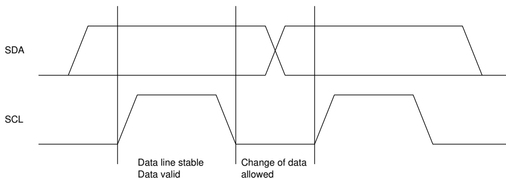
图 6-6. I 2 C 数据有效性
