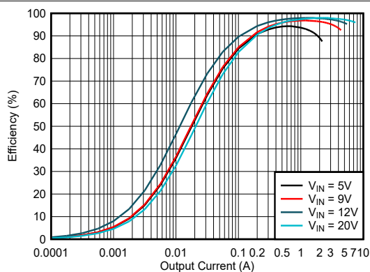
图 5-7. 效率与输出电流间的关系, V_{OUT} = 15V , FPWM
