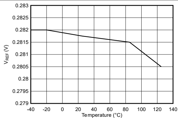
图 5-11. 基准电压与温度间的关系 ( V_{REF} = 0.282V )
