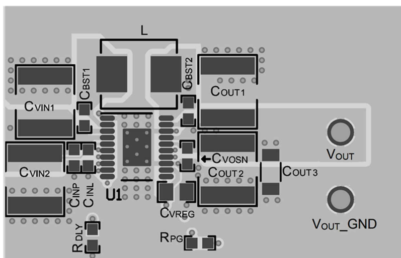
图 11-1. Example Circuit Layout
