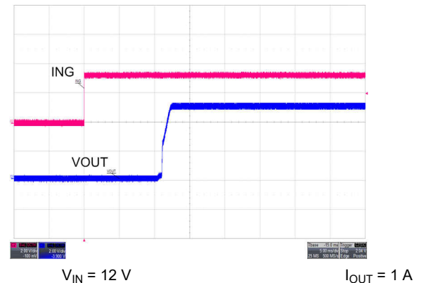
图 9-7. Start-Up Procedure
