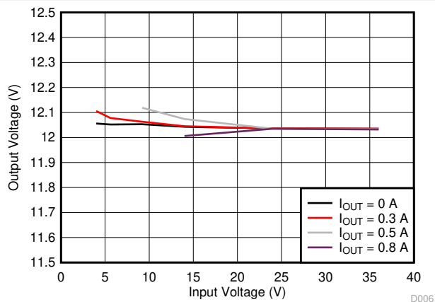
图 7-6. 12-V Output Regulation vs Input Voltage
