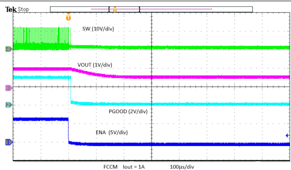
图 8-15. Prebias Power-Down
