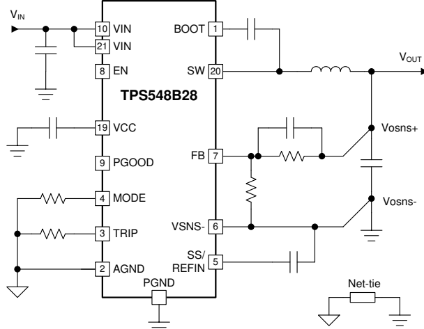
简化原理图
