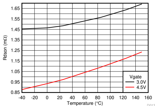
图 6-13. 低侧 MOSFET 导通电阻 ( R_{DS(on)} ) 与结温间的关系
