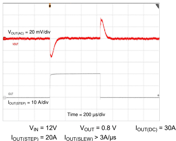
图 8-16. 负载瞬态响应
