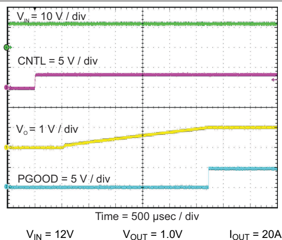
图 8-5. 从 EN/UVLO 启动
