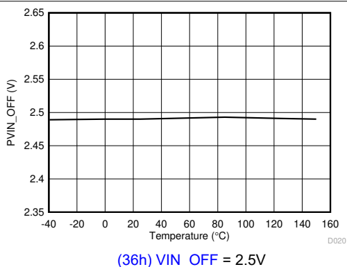
图 6-21. 关断电压与结温间的关系
