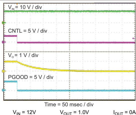
图 8-7. 通过 CNTL 关闭
