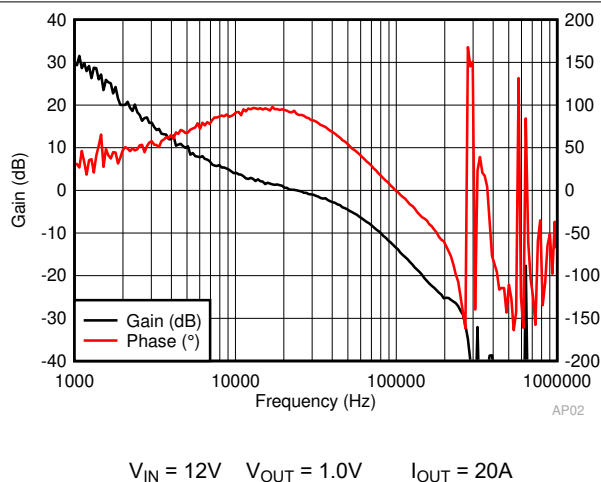
图 8-4. 总环路波特图
