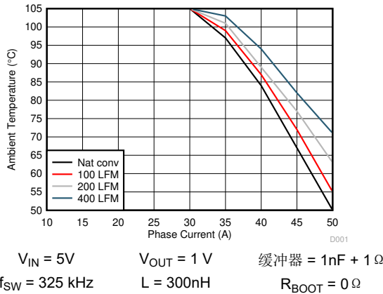
图 6-1. TPS546D24A 安全操作区域
