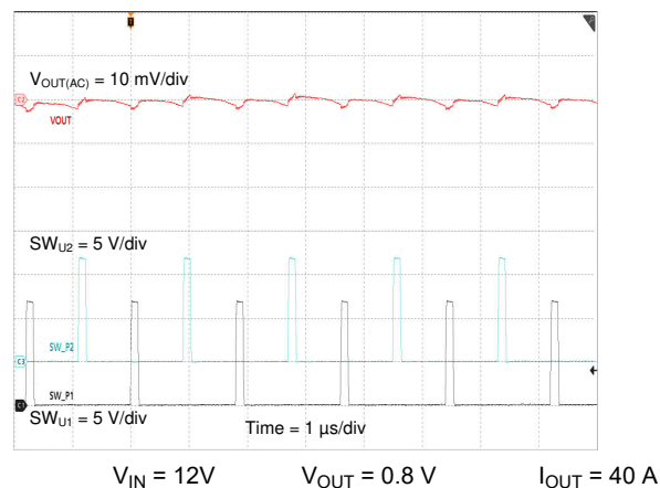
图 8-17. V_{OUT} 稳态纹波
