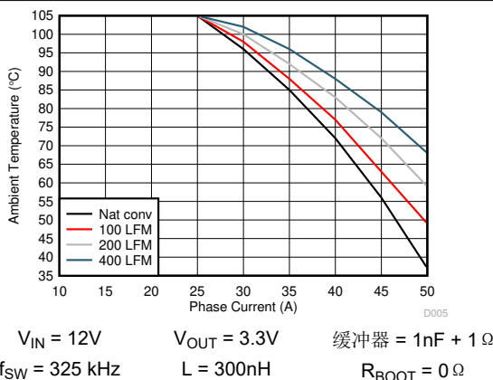
图 6-5. TPS546D24A 安全操作区域
