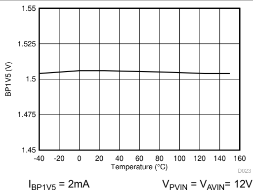
图 6-19. BP1V5 电压与结温间的关系
