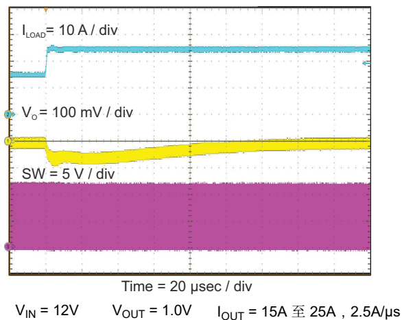
图 8-8. 负载瞬态响应
