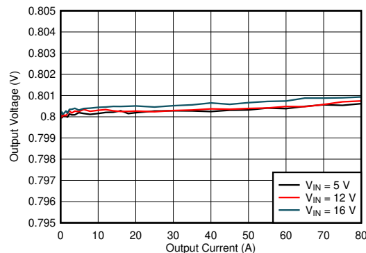
图 8-13. 负载调整率
