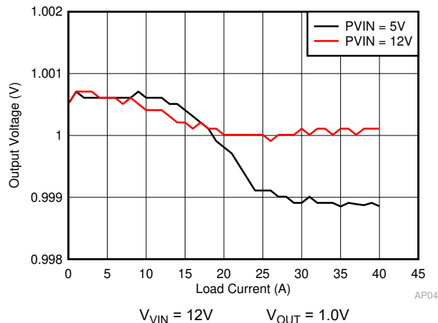
图 8-3. 负载调整率
