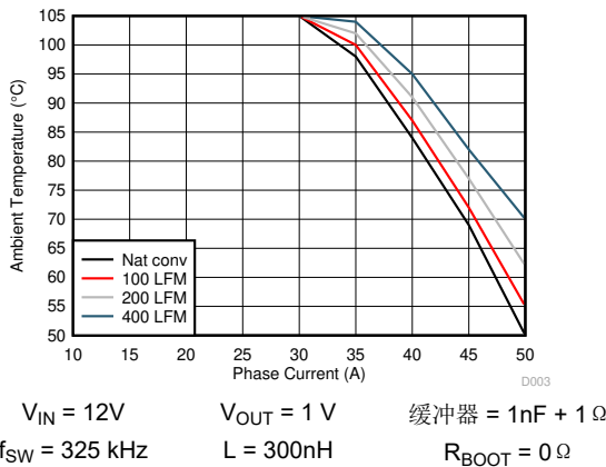
图 6-3. TPS546D24A 安全操作区域
