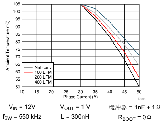
图 6-4. TPS546D24A 安全操作区域
