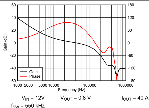
图 8-15. 总环路波特图
