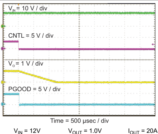
图 8-6. 通过 CNTL 关闭
