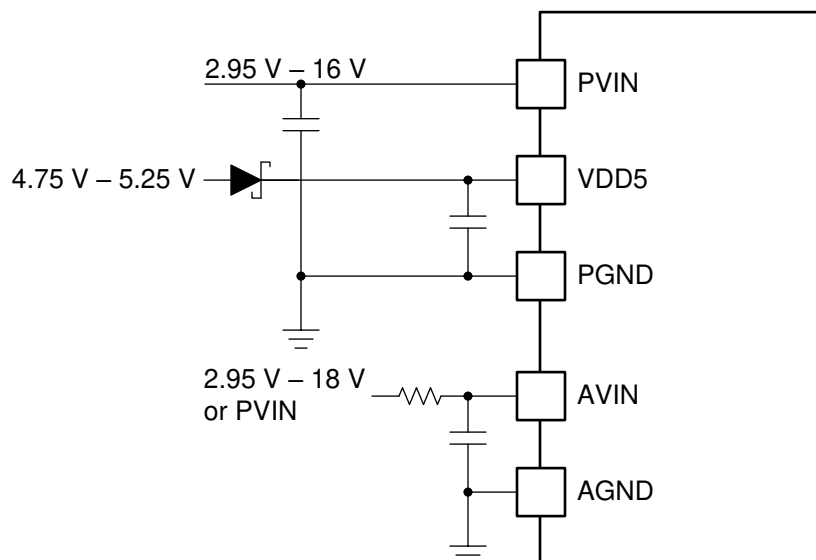
图 7-4. TPS546D24A 单独的 PVIN、AVIN 和 VDD5 连接
