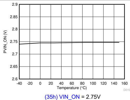
图 6-20. 导通电压与结温间的关系
