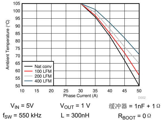
图 6-2. TPS546D24A 安全操作区域
