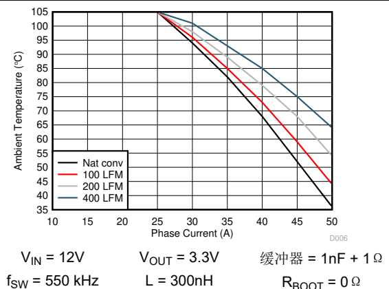
图 6-6. TPS546D24A 安全操作区域
