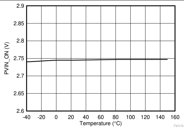
VIN\_ON = 2.75V 图 5-13. 导通电压与结温间的关系
