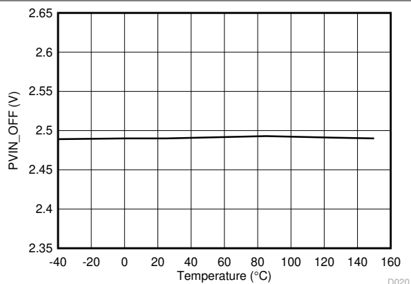
VIN\_OFF = 2.5V 图 5-14. 关断电压与结温间的关系
