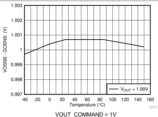
图 5-8. 输出电压与结温间的关系
