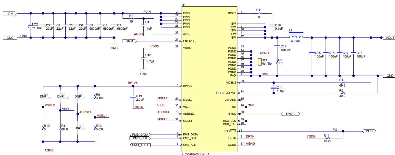
图 7-1. TPS546A24S 应用
