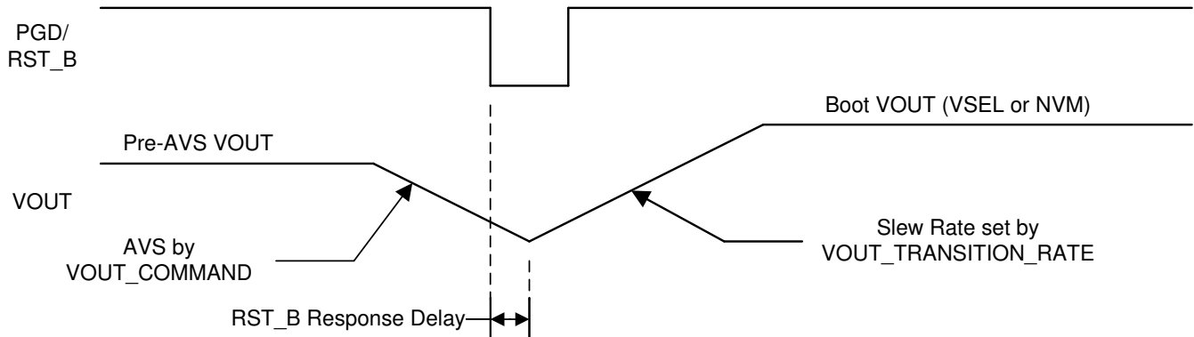
图 6-7. TPS546A24S 输出电压复位
