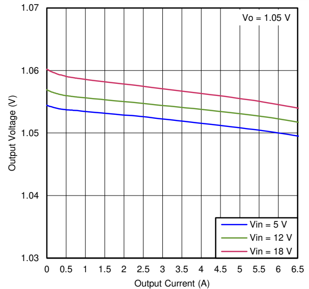
图 12-4. 1.05-V OUTPUT VOLTAGE vs OUTPUT CURRENT
