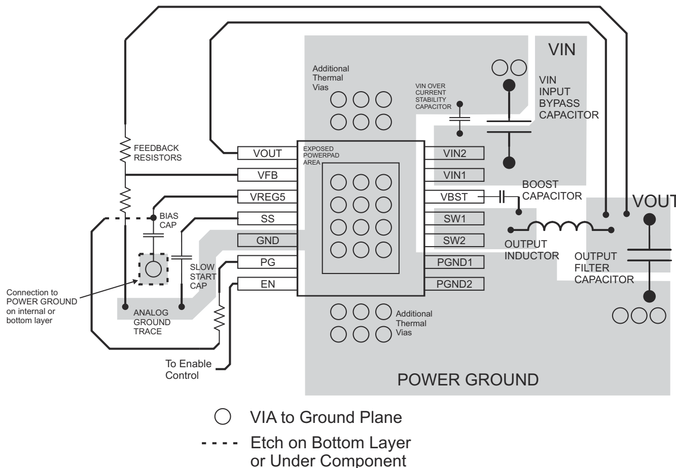
图 15-1. PCB Layout
