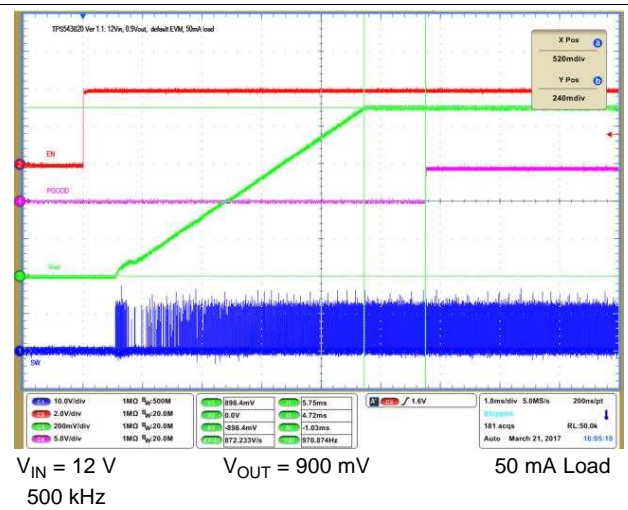
图 10. Startup From EN
