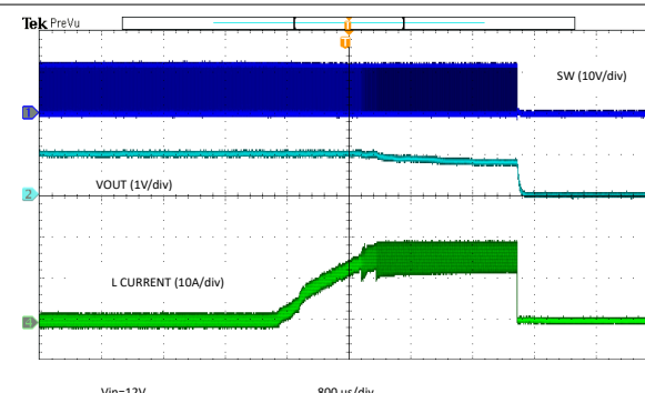
图 7-21. 过流保护 - 短路
