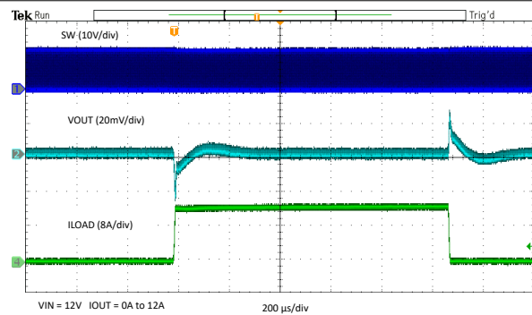
图 7-8. 负载瞬态
