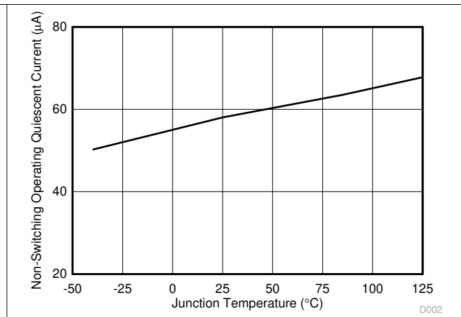
图 5-2. 非开关工作静态电流与结温间的关系
