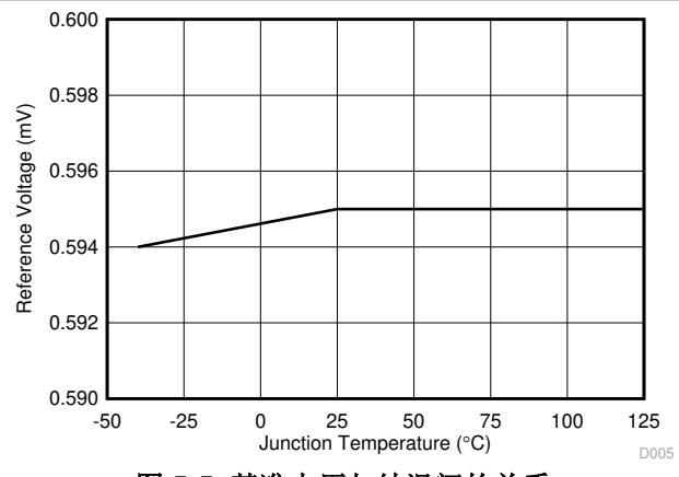
图 5-5. 基准电压与结温间的关系
