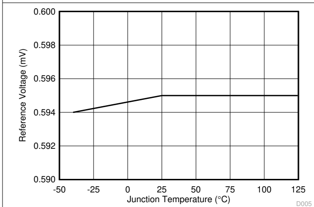
图 5-5. 基准电压与结温间的关系
