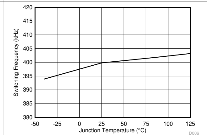
图 5-6. 中心开关频率与结温间的关系
