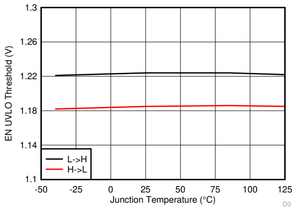
图 5-11. EN 阈值与结温间的关系
