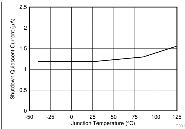
图 5-1. 关断静态电流与结温间的关系
