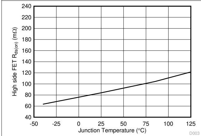
图 5-3. 高侧电阻与结温间的关系
