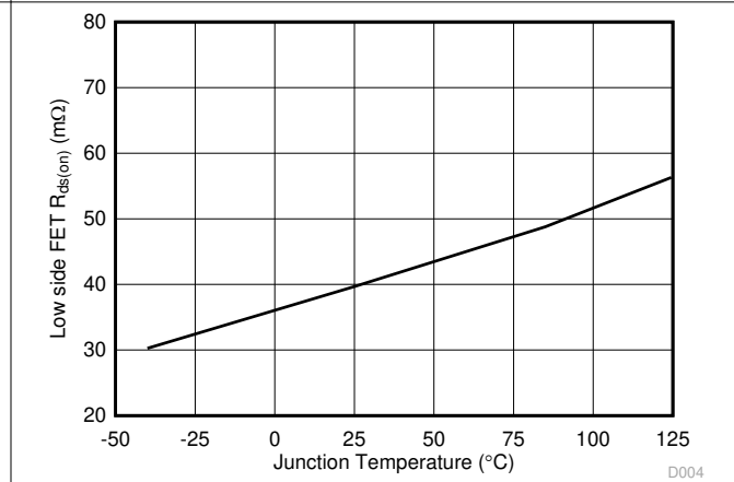
图 5-4. 低侧 FET 导通电阻与结温间的关系
