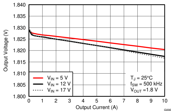
图 9-14. Load Regulation
