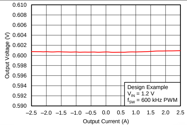
图 36. Load Regulation
