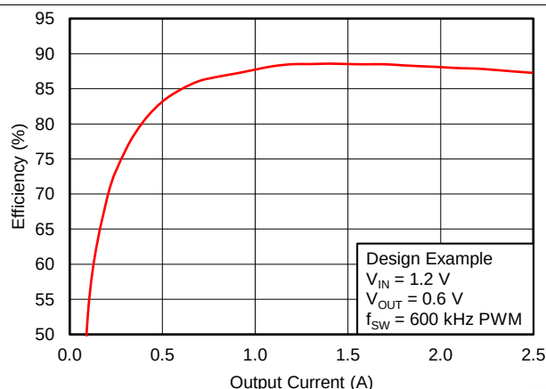
图 31. Efficiency
