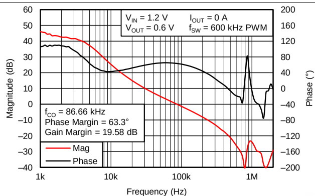
图 33. Bode Plot, No Load
