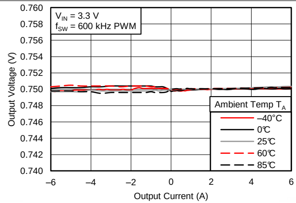
图 12. Load Regulation
