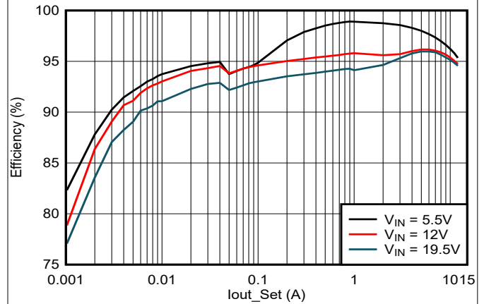
图 5-16. 效率与负载电流间的关系, 560kHz, Eco-mode
