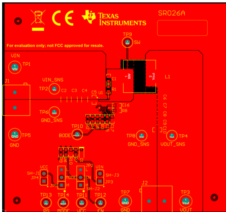
图 7-20. 顶面布局
