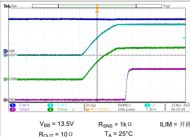
图 6-14. 开关导通
